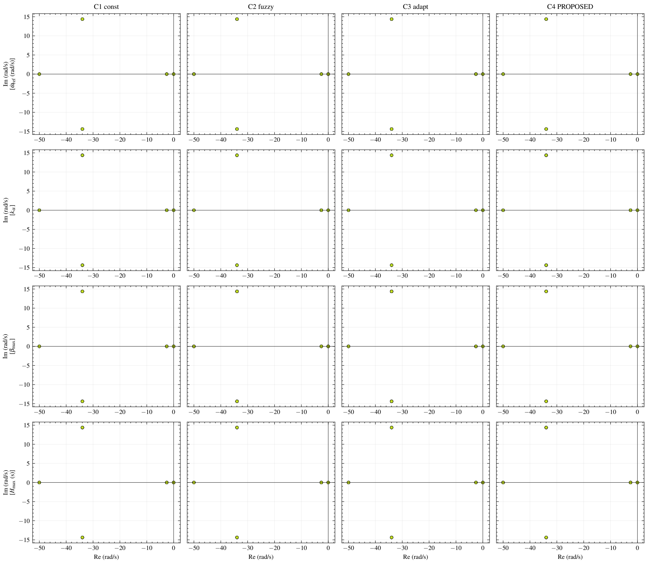
Eigenvalue locus on s -plane — sweep 4 parameters \times 4 schemes (viridis: low \rightarrow high parameter value)
