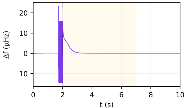
Residual f (Julia - MATLAB)
