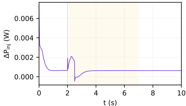
Residual P_{\text{inj}} (Julia - MATLAB)
