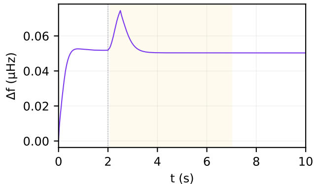
Residual f (Julia - MATLAB)
