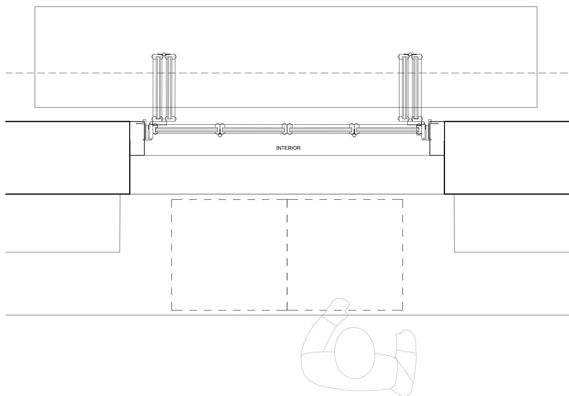
X BAR WINDOW - PLAN SCALE: 1" = 1'-0"
