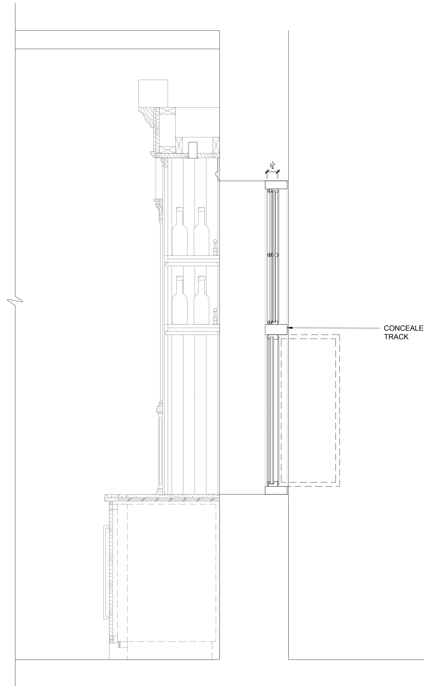
X BAR WINDOW - SECTION SCALE: 1" = 1'-0"
