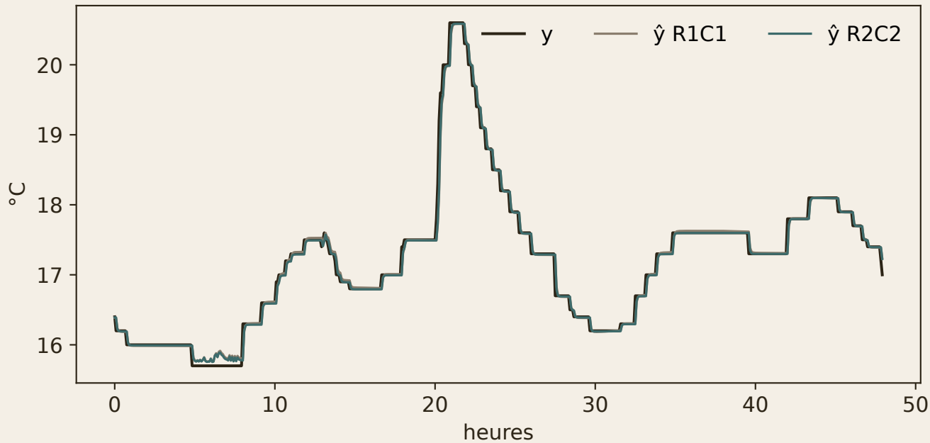
48 h autour d'un pic PV (test)
