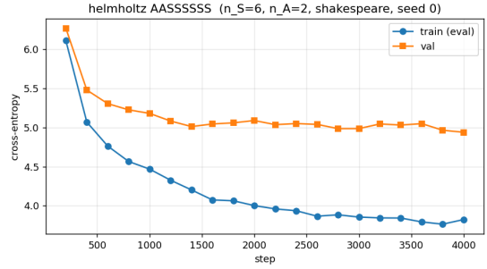
(b) Q9d AASSSSSS vh=128 seed 0, val PPL 139.63.
