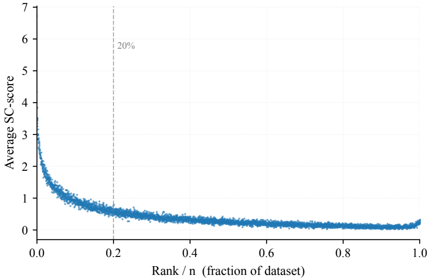
SIFT10M
