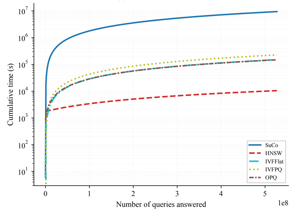
(d) SIFT10M, Recall \geq 0.9
