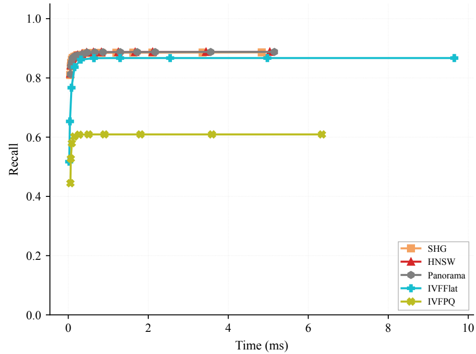
UQ-V (k=20)
