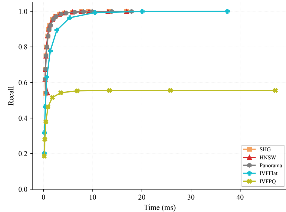
MsTuring10M (k=20)
