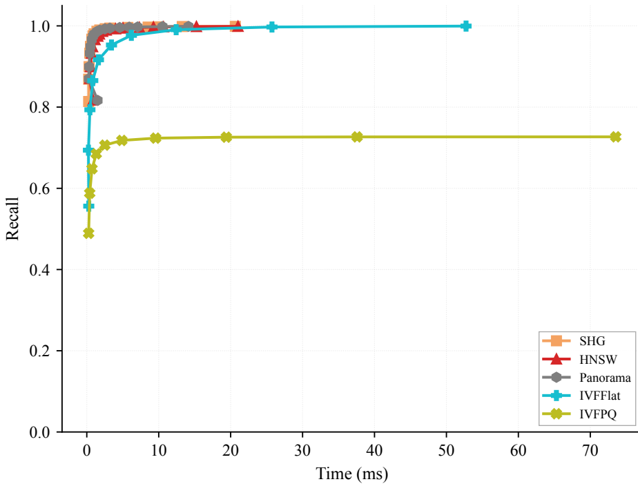
Msong (k=20)
