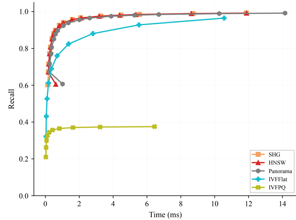
MsTuring10M (k=20)
