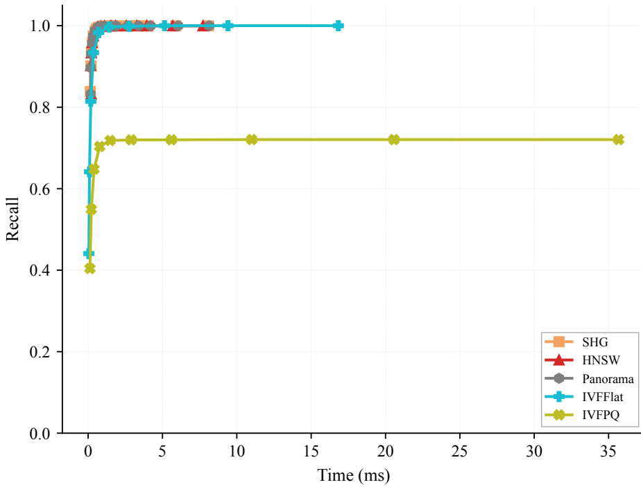
Msong (k=20)
