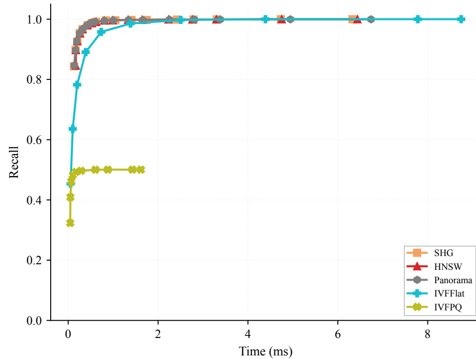
UQ-V (k=20)
