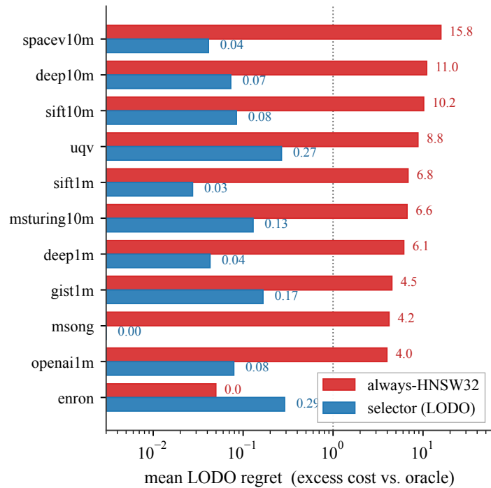
(b) per held-out dataset
