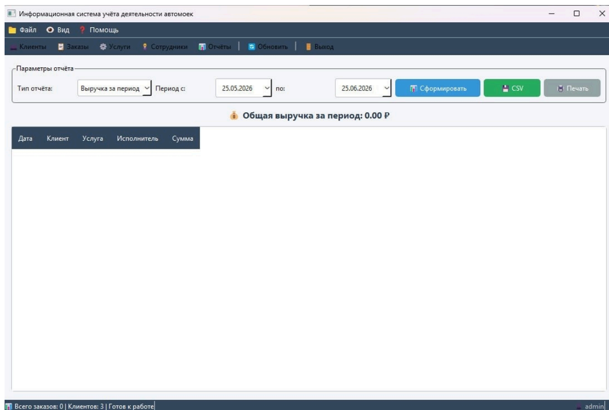
Рисунок 7. Раздел «Отчёты»
