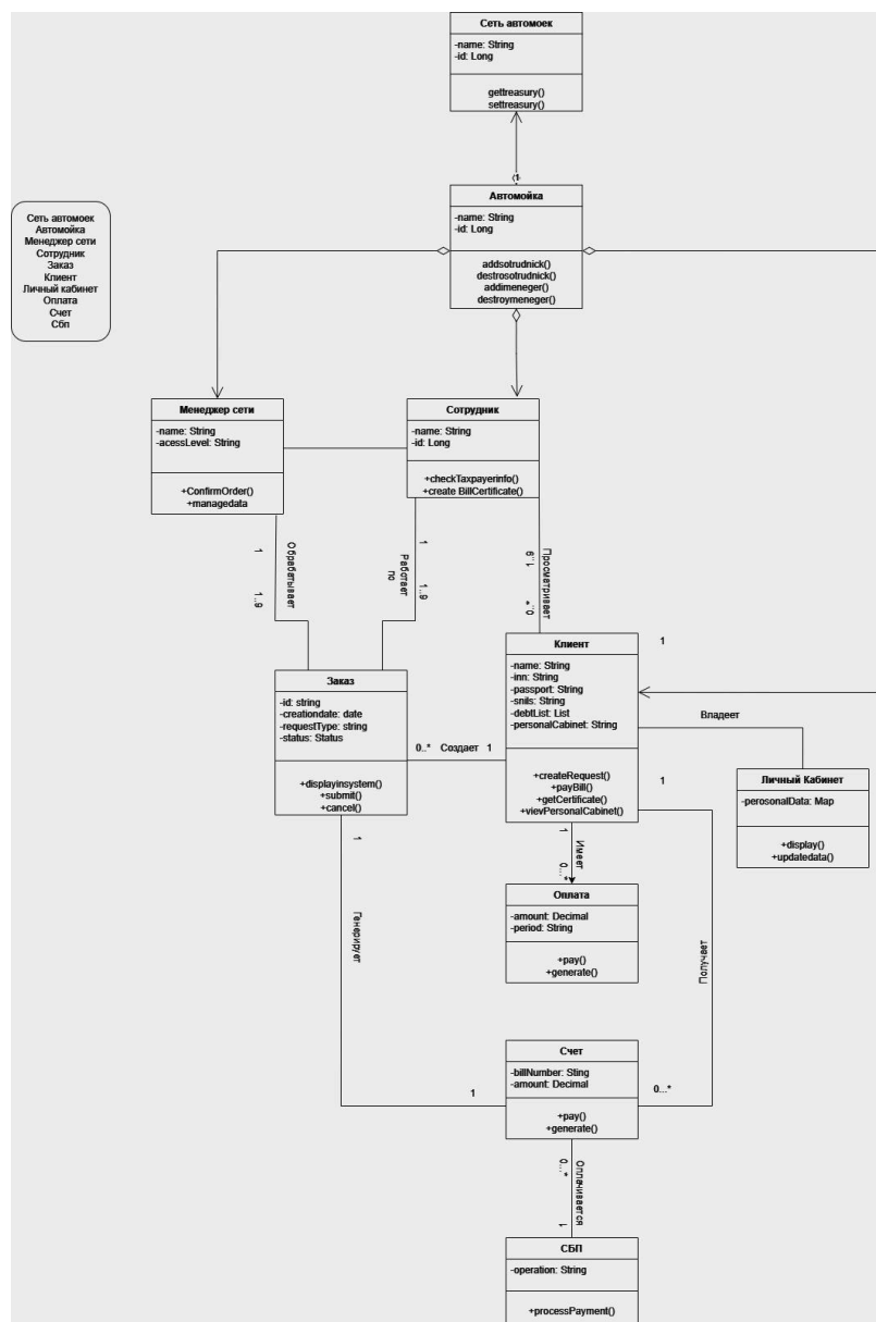
Рисунок 9. Диаграмма классов
