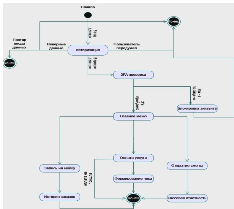
Рисунок 2. Диаграмма деятельности
