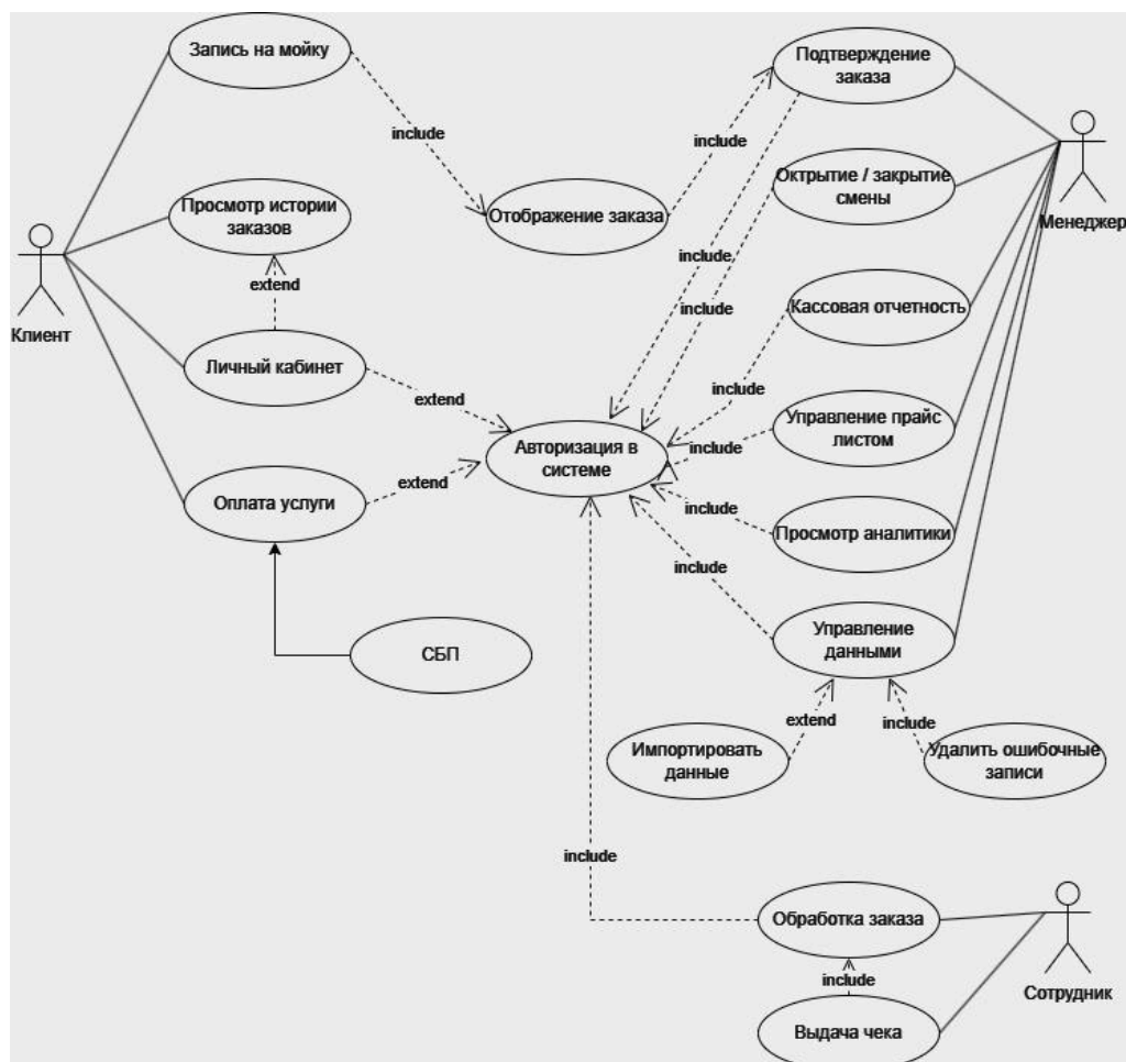
Рисунок 8. Диаграмма вариантов использования
