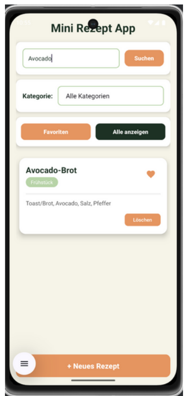
Bild 11: Startseite - Einwortsuche "Avocado"
