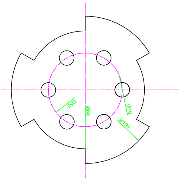
密封垫
