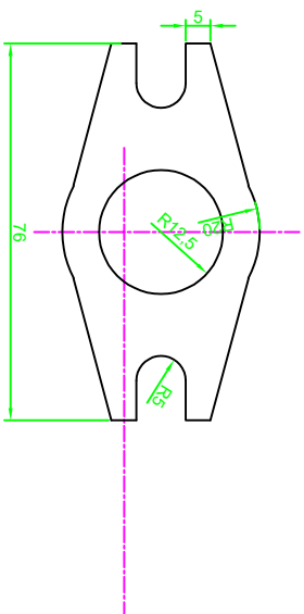
卡盘
