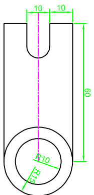
支架
