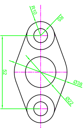
压盖
