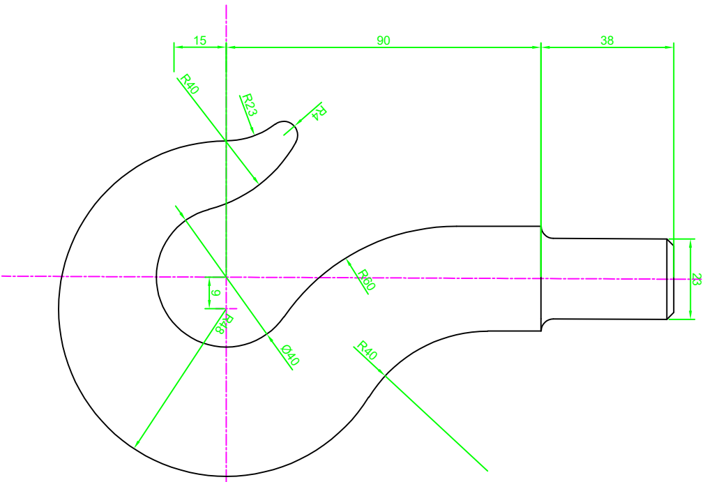
起重钩
