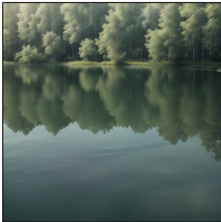
PSDiffusion (Ours)
