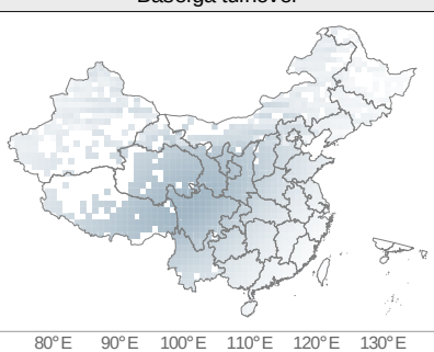
Baselga turnover
