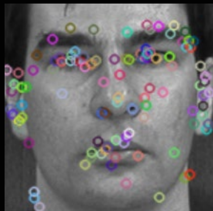
Sift
