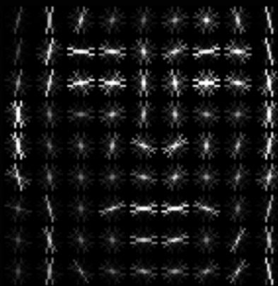
Hog
