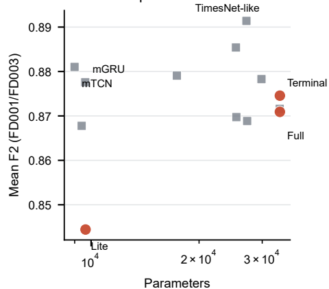
C-MAPSS parameter count vs F2
