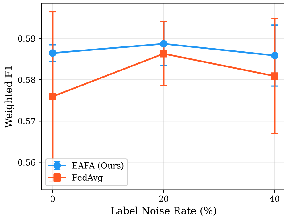
IEMOCAP
