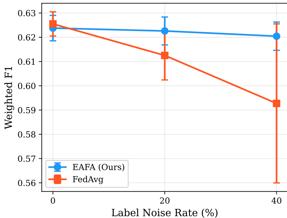
MELD
