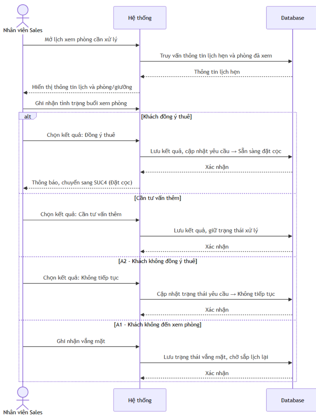
Figure 36: Sơ đồ tuần tự – SUC15: Ghi nhận kết quả xem phòng
