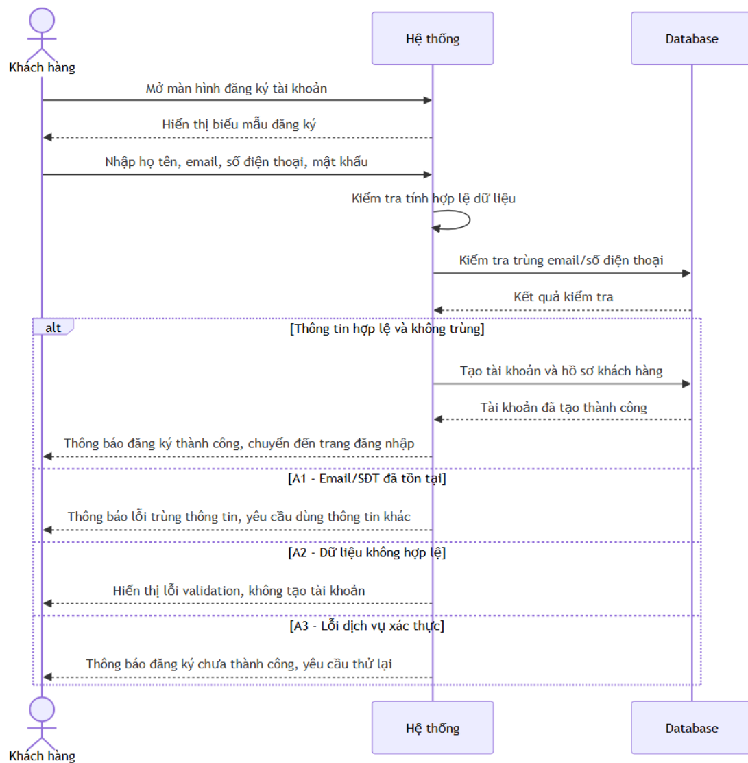
Figure 39: Sơ đồ tuần tự – SUC18: Đăng ký tài khoản khách hàng
