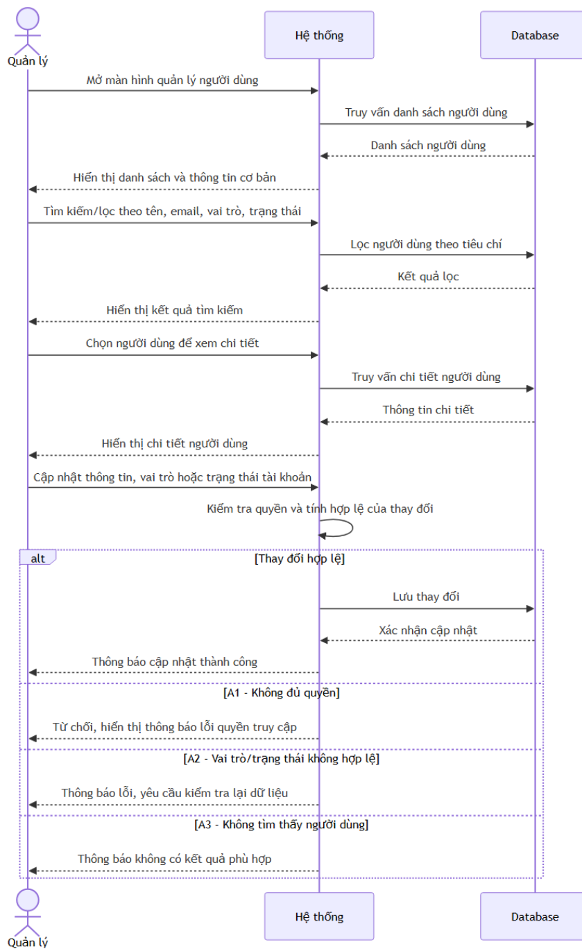
Figure 40: Sơ đồ tuần tự – SUC19: Quản lý người dùng
