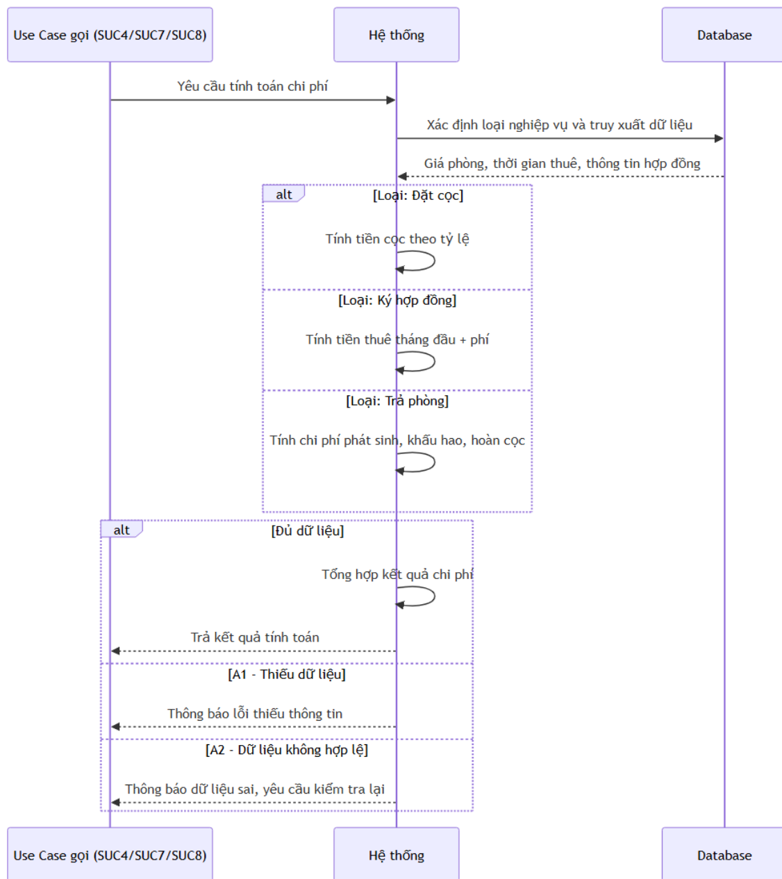
Figure 30: Sơ đồ tuần tự – SUC9: Tính toán chi phí
