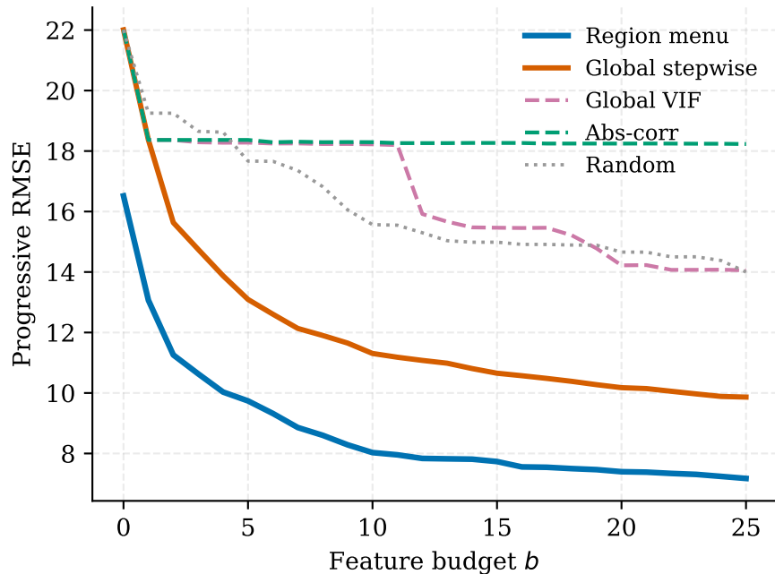
CT slices ( n=8\{, \}000 , p=384 )
