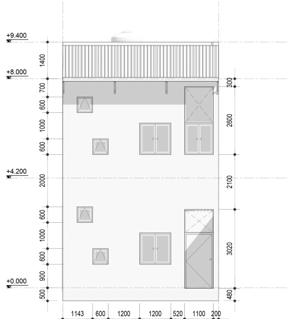
MẶT ĐÚNG 1-2
