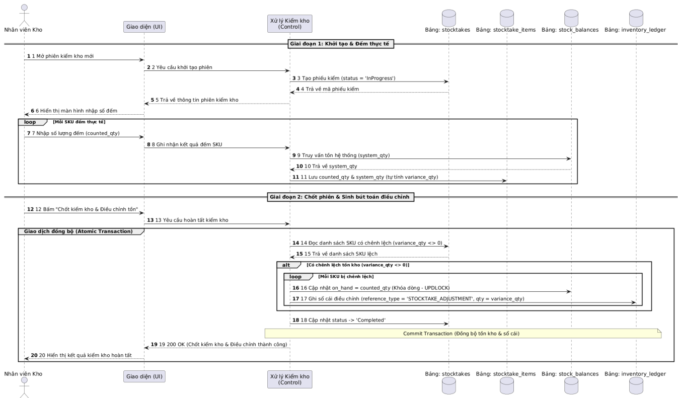
Hình 3.7: Sequence Diagram — luồng kiểm kho & sinh bút toán điều chỉnh
