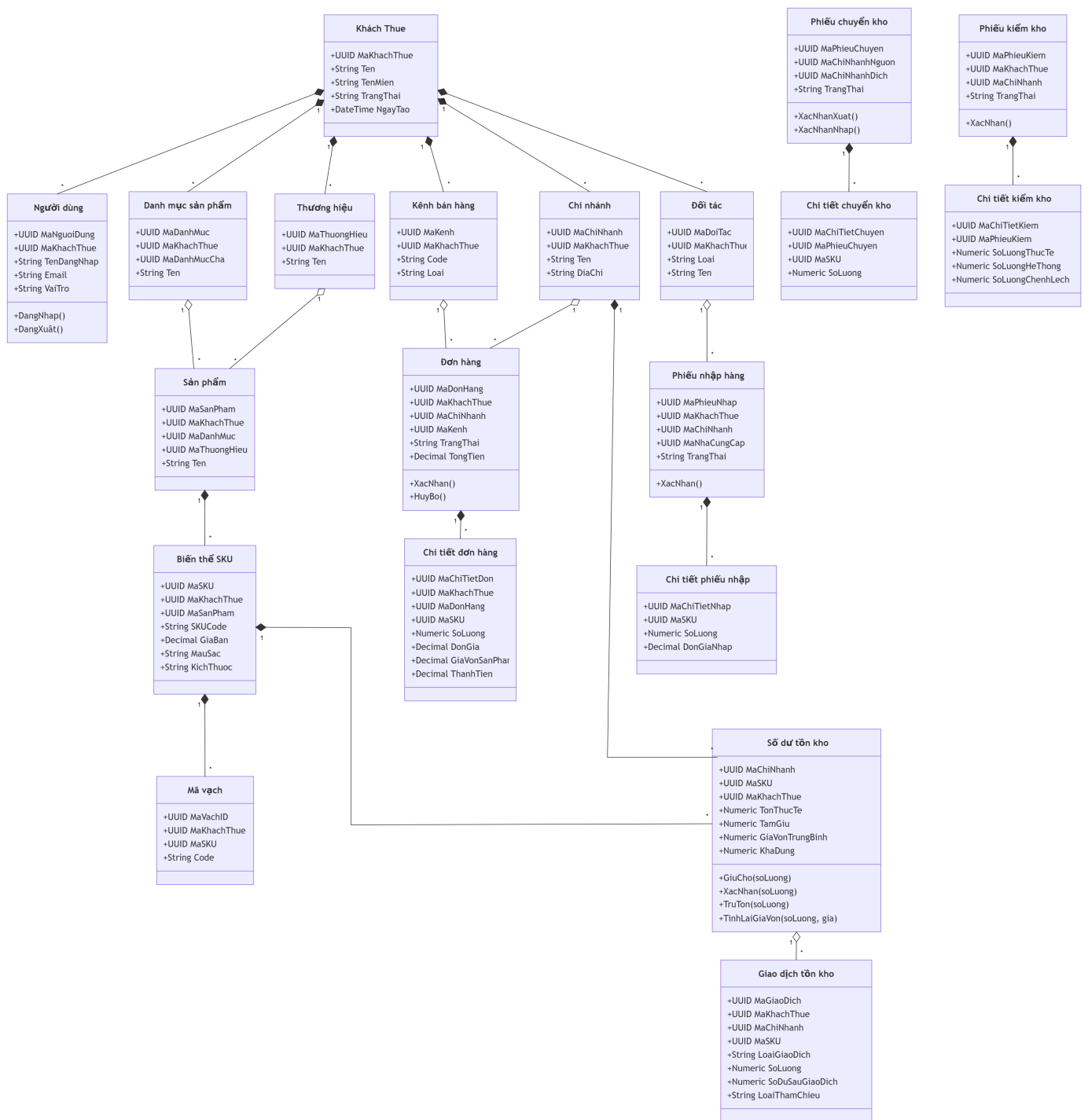
Hình 3.4: UML Class Diagram các entity chính
