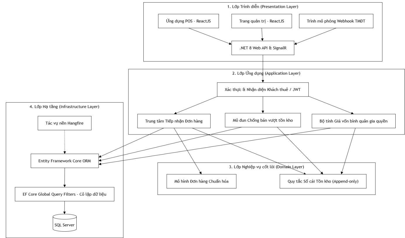
Hình 3.1: Sơ đồ kiến trúc tổng thể hệ thống (Architecture / System Context Diagram)
