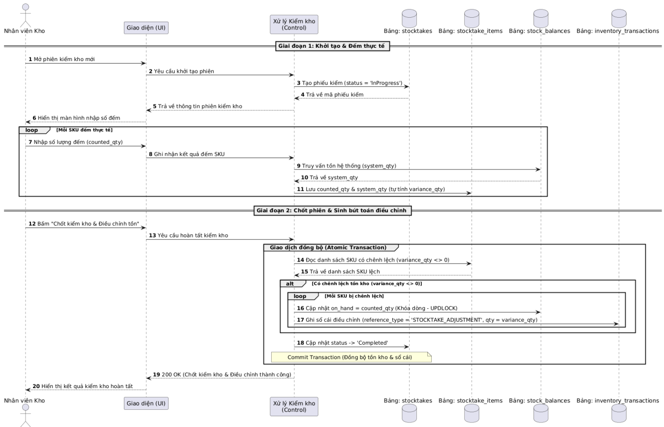
Hình 3.7: Sequence Diagram — luồng kiểm kho &amp; sinh bút toán điều chỉnh
