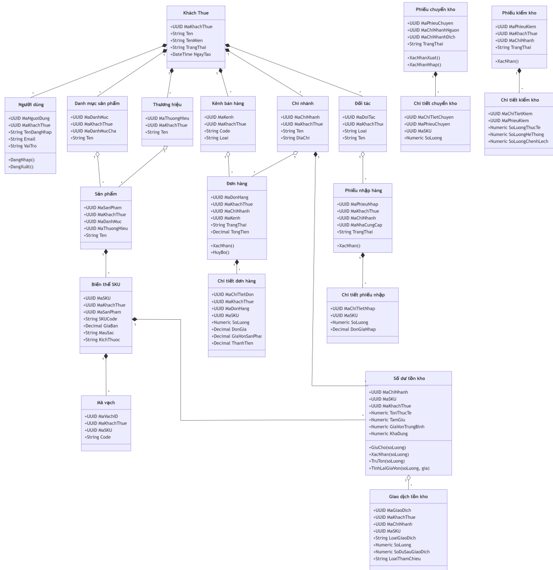
Hình 3.4: UML Class Diagram các entity chính
