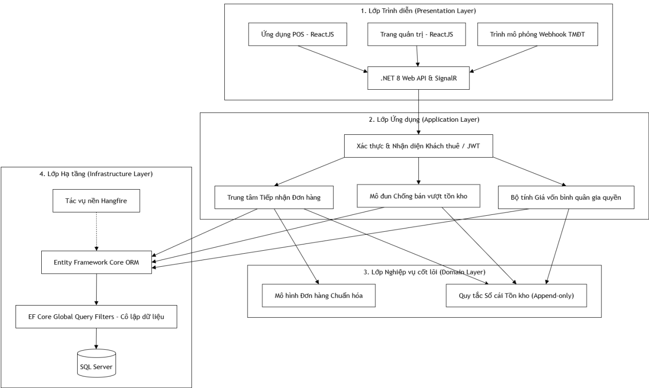
Hình 3.1: Sơ đồ kiến trúc tổng thể hệ thống (Architecture / System Context Diagram)
