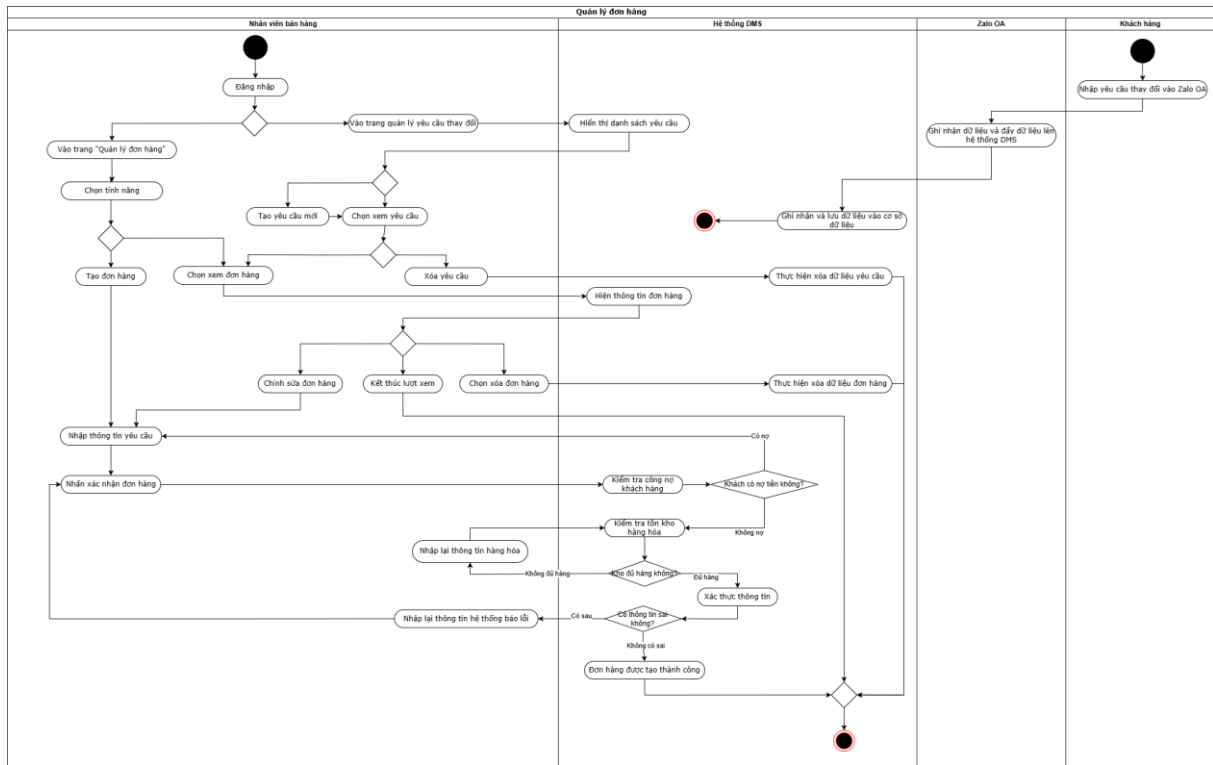
Hình 5.13: Activity Diagram mô tả hoạt động quản lý đơn hàng Link
