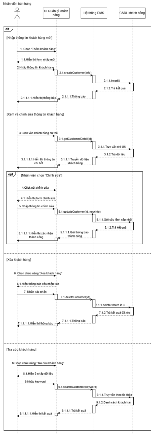
Hình 5.8: Sequence diagram 2 - Quản lý khách hàng Link
