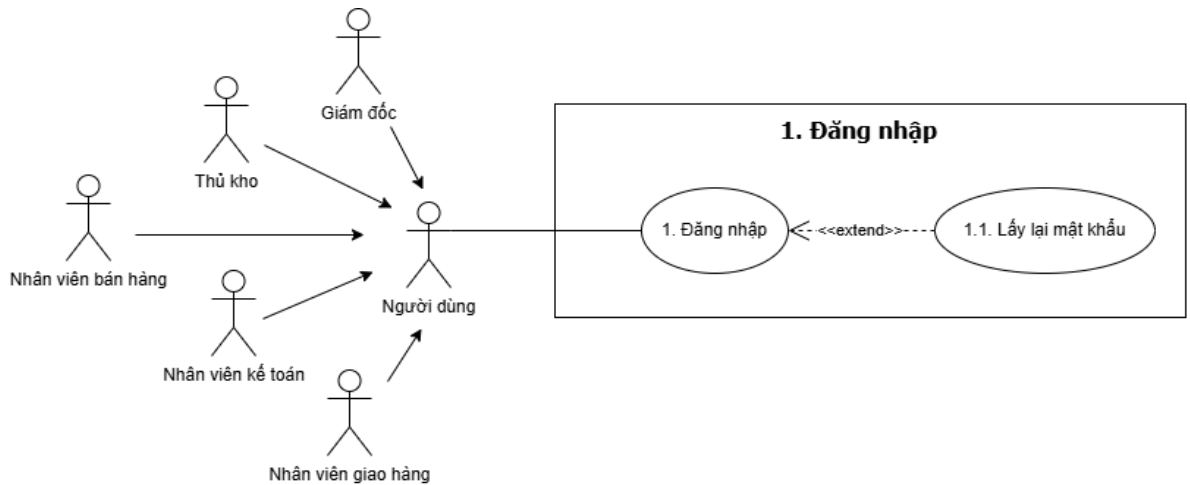
Hình 5.3: Mô tả Use Case 1 - Đăng nhập
