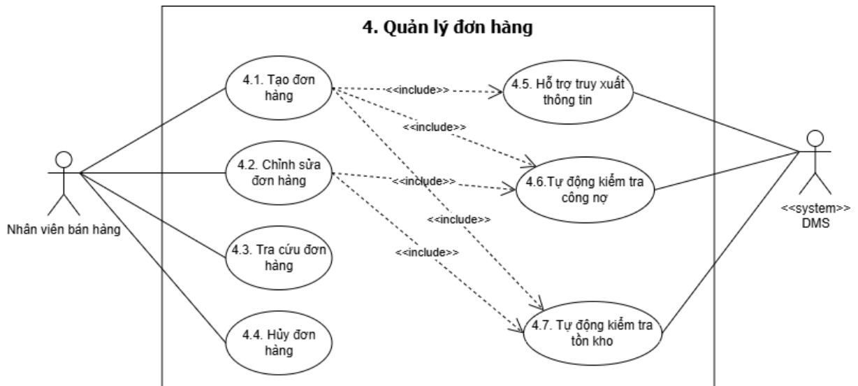
Hình 5.12: Mô tả Use Case 4 – Quản lý đơn hàng
