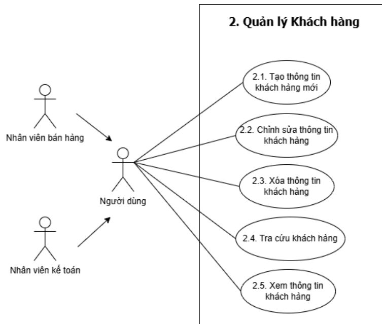
Hình 5.6: Mô tả Use Case 2 – Quản lý khách hàng
