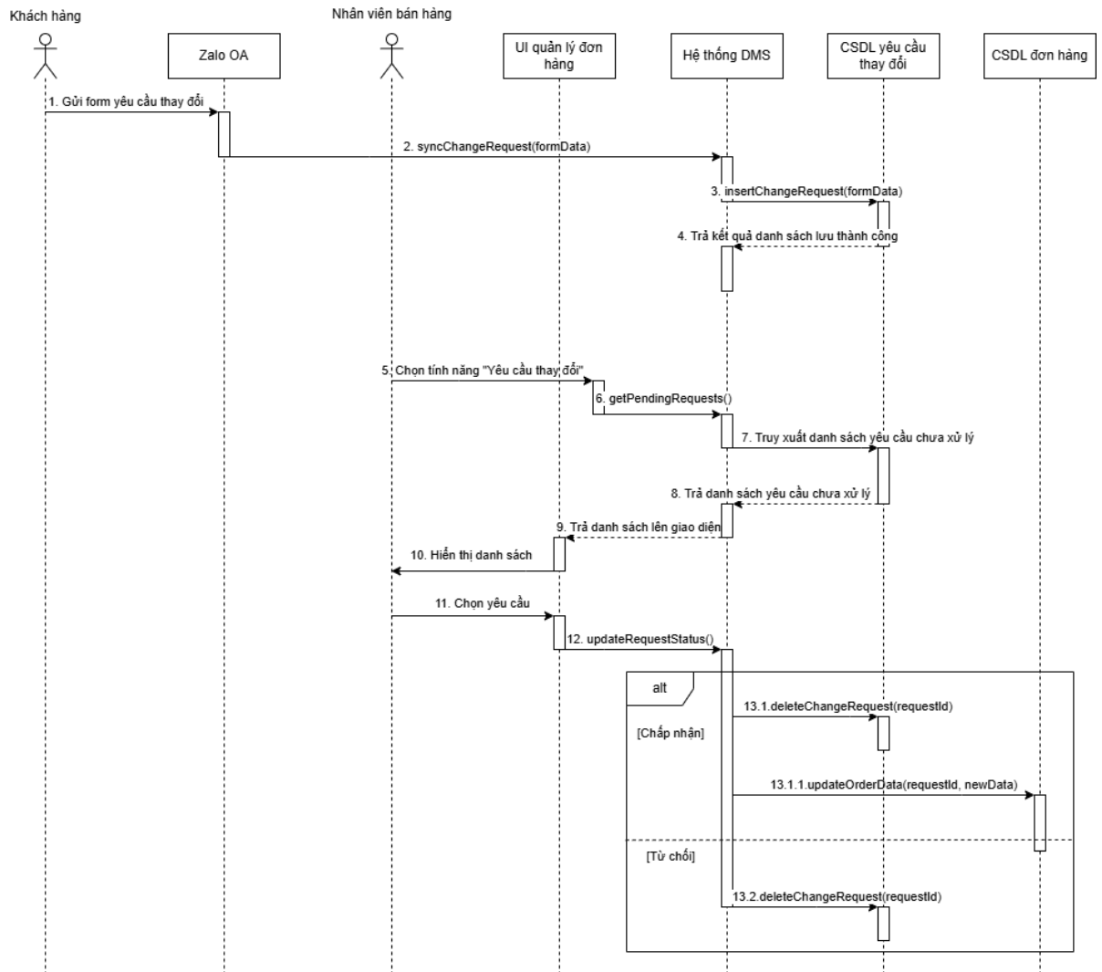
Hình 5.19: Sequence diagram 6 - Quản lý yêu cầu thay đổi Link
