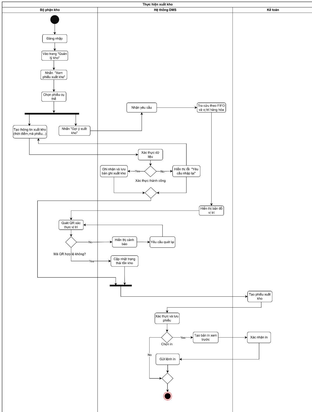
Hình 5.16: Activity Diagram mô tả hoạt động thực hiện xuất kho Link
