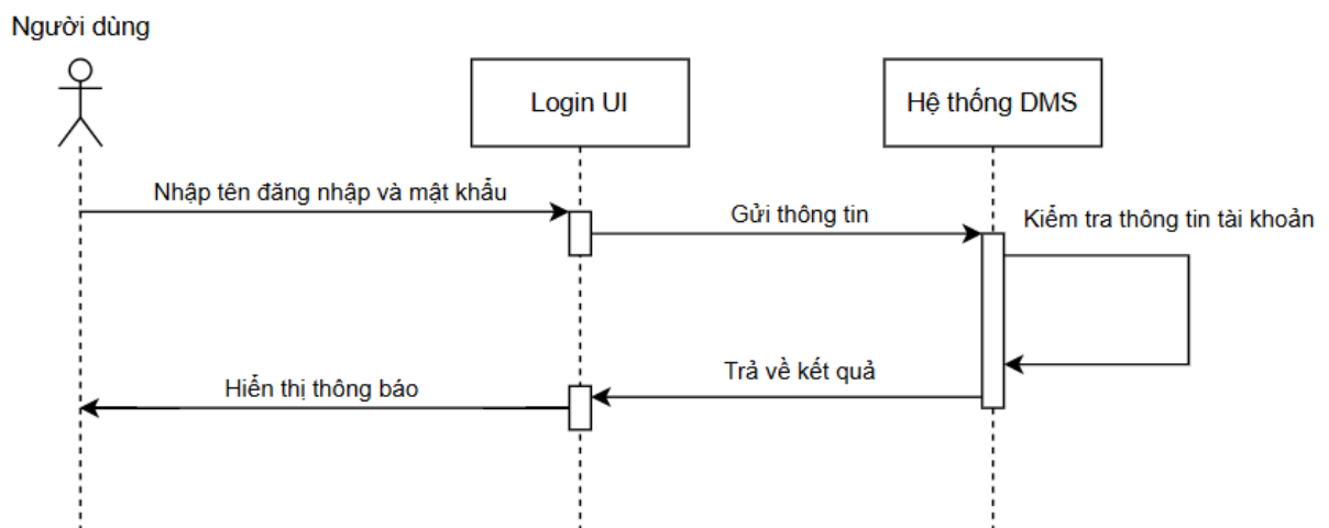
Hình 5.5: Sequence diagram 1 - Đăng nhập
