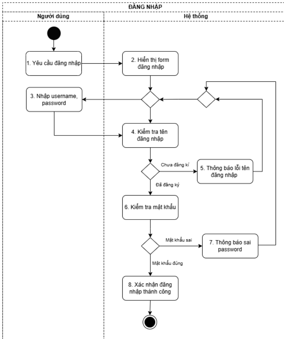
Hình 5.4: Activity Diagram mô tả hoạt động đăng nhập
