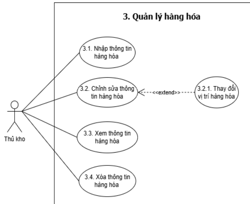
Hình 5.9: Mô tả Use Case 3 – Quản lý hàng hóa
