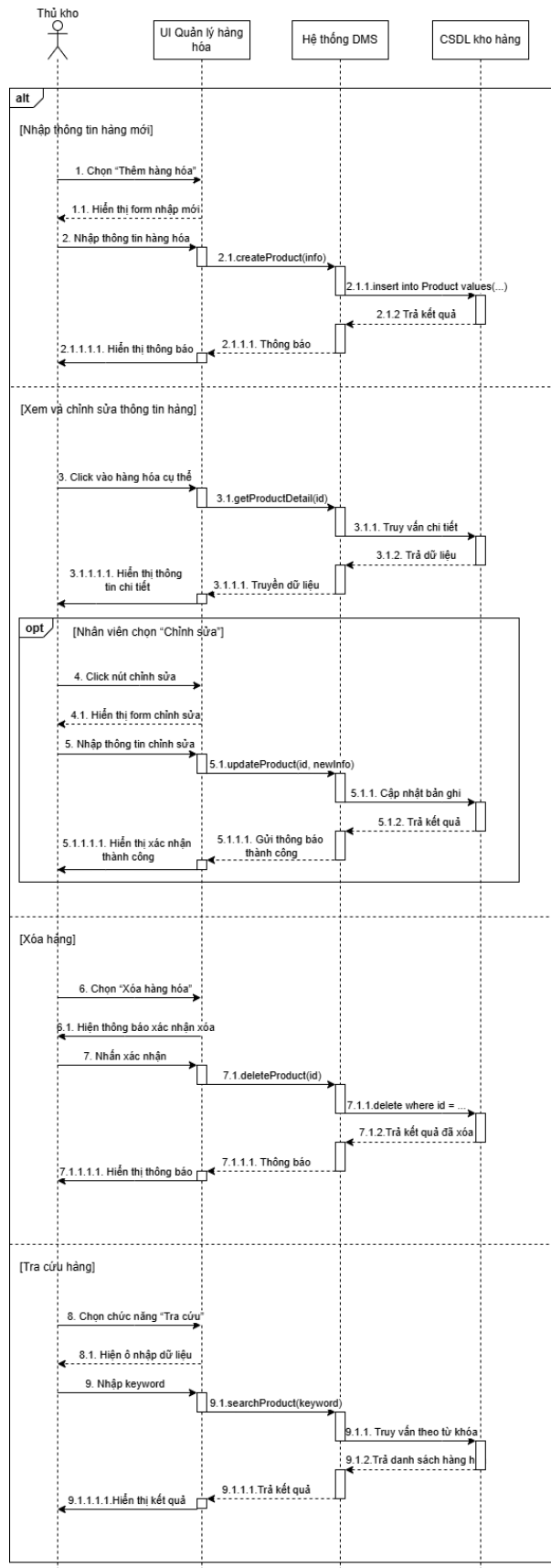
Hình 5.11: Sequence diagram 3 - Quản lý hàng hóa Link
