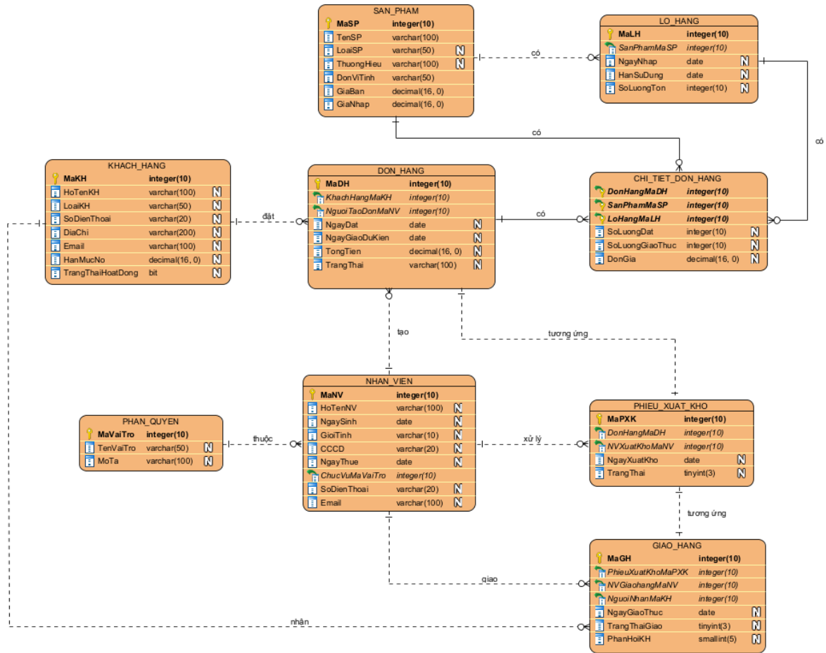
Hình 5.21: Mô hình ERD
