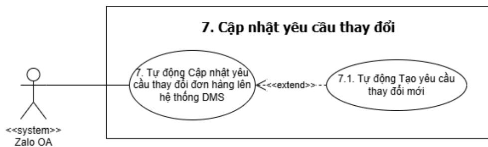
Hình 5.20: Mô tả Use Case 7 – Cập nhật yêu cầu thay đổi
