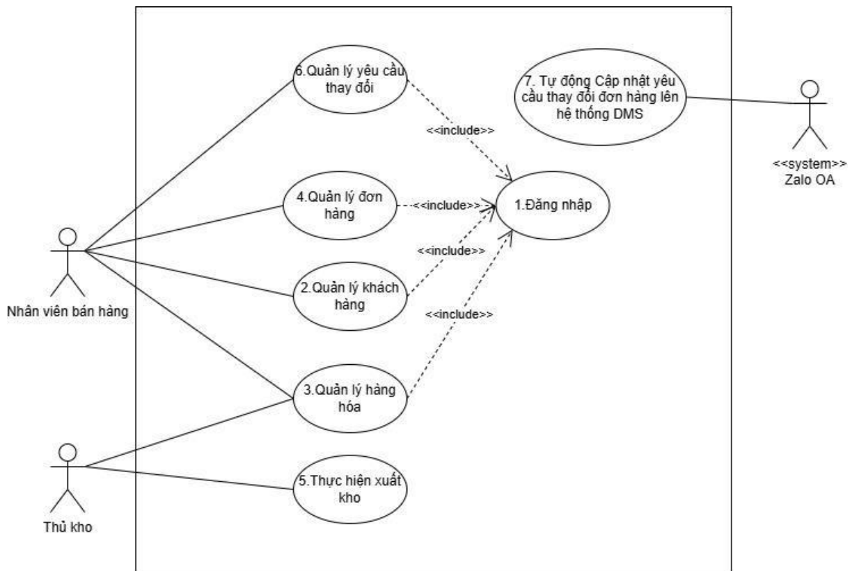
Hình 5.2: Mô tả Use Case tổng quát
