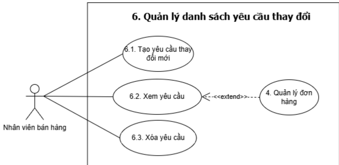
Hình 5.18: Mô tả Use Case 6 – Quản lý danh sách yêu cầu thay đổi
