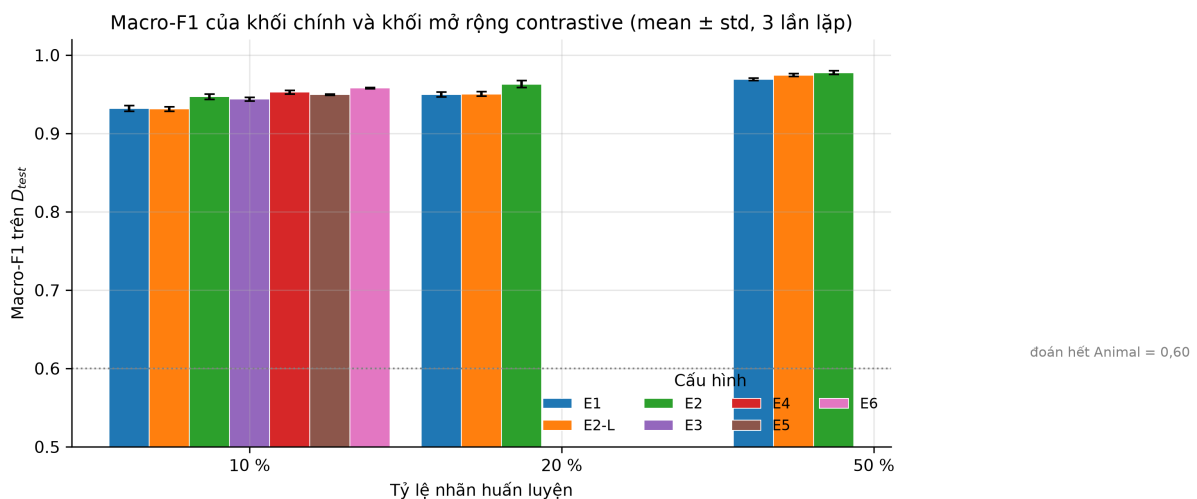
Hình 11: Macro-F1 trên D_{\text{test}} của các cấu hình đã có kết quả, trung bình qua các lần lặp đã xong, so với mức 0,60 của bộ phân loại luôn đoán Animal. Khối chính (E1, E2-L, E2) có kết quả ở cả ba mức nhấn; khối mở rộng contrastive chỉ được khảo sát ở mức 10 % nhấn (xem Bảng 21). Hình được sinh lại tự động bởi scripts/make_extension_figures.py, nên số cột phản ánh đúng số cấu hình đã chạy xong tại thời điểm sinh báo cáo.
