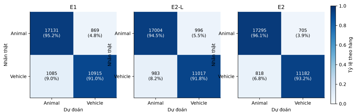
Hình 8: Ma trận nhầm lẫn trên D_{\text{test}} tại mức 10 % nhân, gộp ba lần lặp (tổng 30.000 dự đoán cho mỗi cấu hình). Ô ghi số lượng tuyệt đối và tỷ lệ theo hàng. Ma trận cho thấy phần lớn sai số tập trung ở lớp Vehicle bị dự đoán thành Animal.
