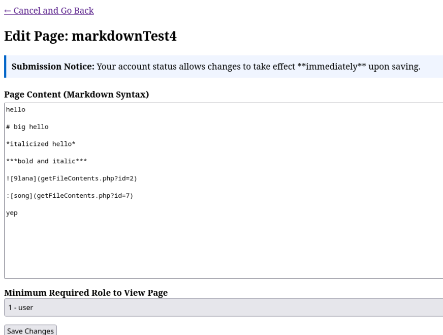
Figura 16 - Editor de página da wiki
