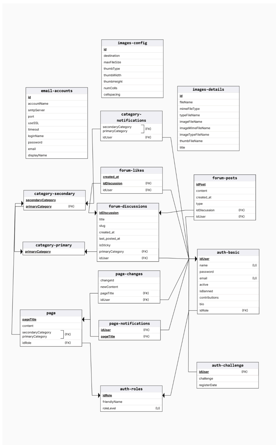
Figura 7 - Modelo relacional da base de dados
