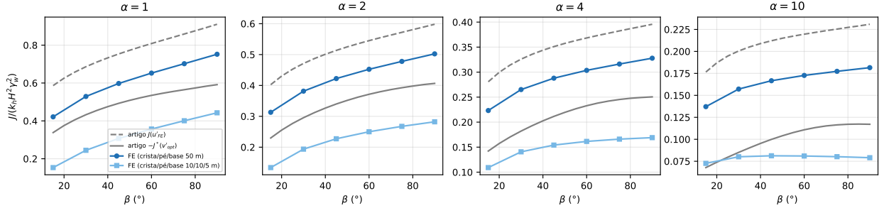
Figura R1: J(u)/(k_h H^2 \gamma_w^2) do FE em poropressão (malha convergida) para dois domínios (crista/pé/base 10/10/5 m e 50/50/50 m), com as estimativas do artigo J(u'_{FE}) (tracejada) e -J^*(\underline{v}'_{opt}) (contínua); só o domínio grande fica entre elas.
