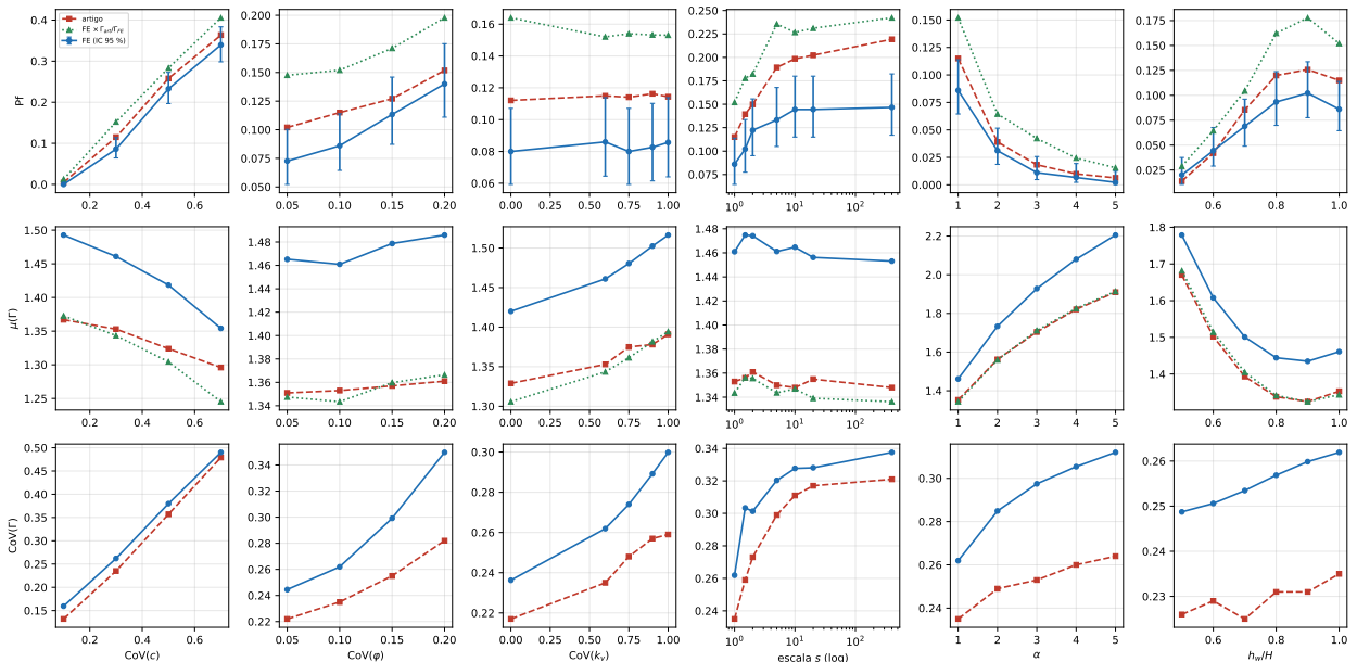
Figura R5: Tendências das Tabelas 3 a 6 do artigo (Tabelas R6 a R9): P_f , \mu(\Gamma) e \text{CoV}(\Gamma) . Vermelho: artigo; azul: FE (barras: IC de 95% de P_f ); verde: FE reescalado. Eixo de s em escala logarítmica.
