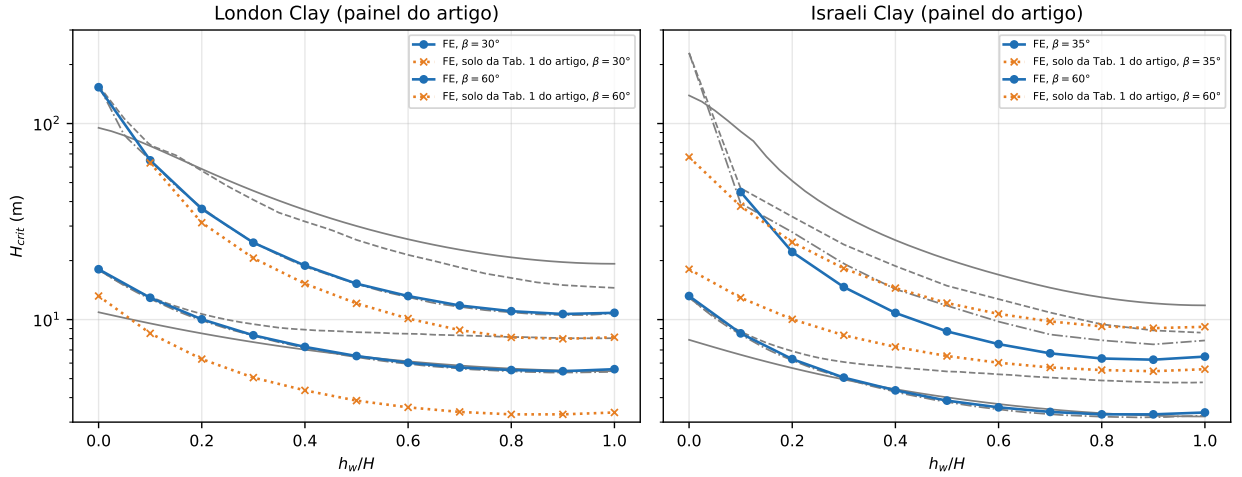
Figura R2: Fig. 8 do artigo (cinza: contínua r_p = 0,25 de Wu et al.; tracejada \underline{K} \cdot \underline{v}'_{opt} ; traço-ponto -\text{grad } u'_{FE} ) e FE (azul: solo que reproduz o artigo em h_w = 0 ; laranja: solo da Tabela 1 do artigo para o rótulo do painel), nível 3.
