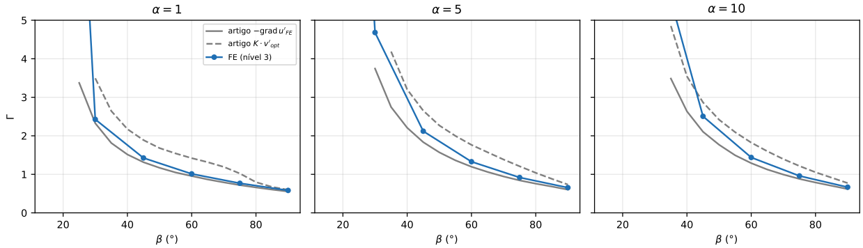
Figura R3: \Gamma \times \beta para \alpha = 1, 5, 10 ( H = h_w = 5 m, c = 10 kPa, \varphi = 30^\circ , \gamma = 20 kN/m 3 ). Cinza: Fig. 9 do artigo (contínua -\text{grad } u'_{\text{FE}} , tracejada \underline{K} \cdot \underline{v}'_{\text{opt}} ). Azul: FE, nível 3, crista 10 m, pé 10 m, base 5 m.
