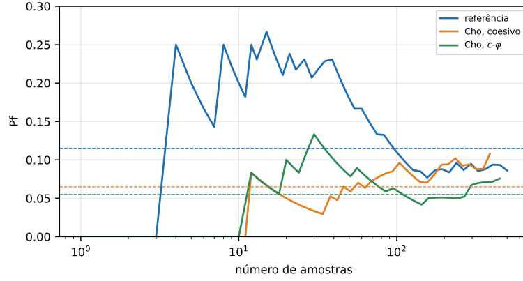
Figura R6: Convergência de Pf com o número de amostras (tracejadas: valores do artigo).
