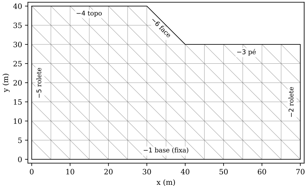
TriGMesh(1): 196 triângulos (P2), talude de 10 m a 45°
