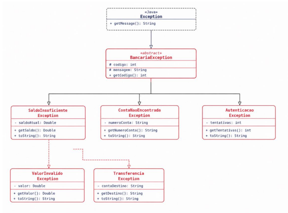
Figura 22 - Diagrama de Classes de Exceções
