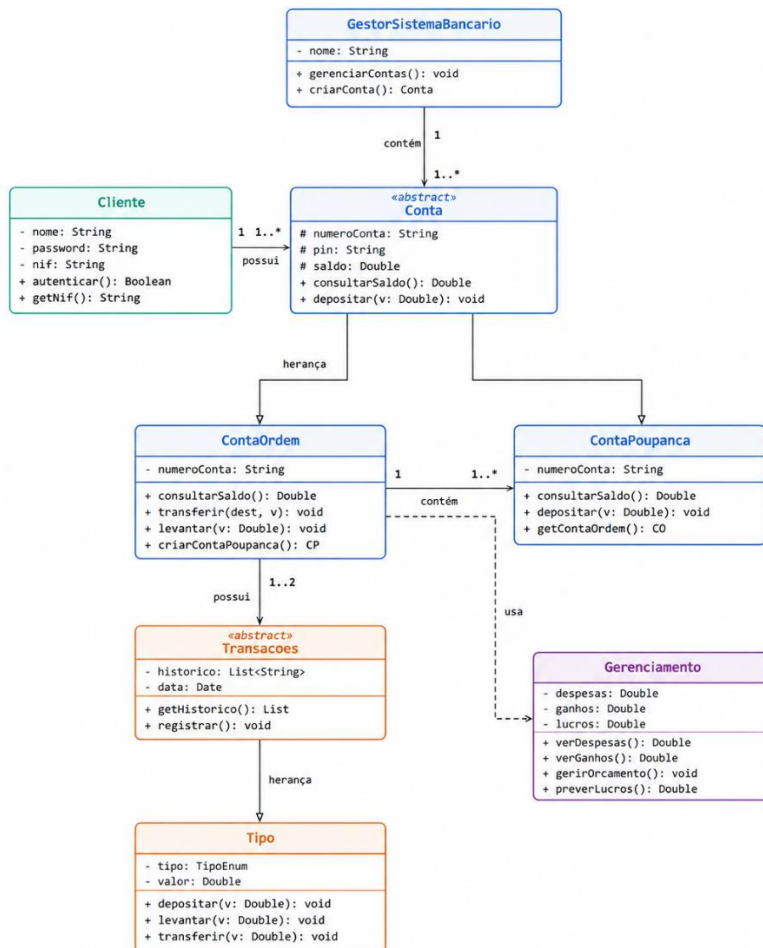
Figura 21 - Diagrama de Classes do Modelo
