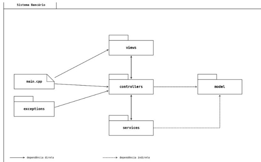
Figura 20 - Organização do Código
