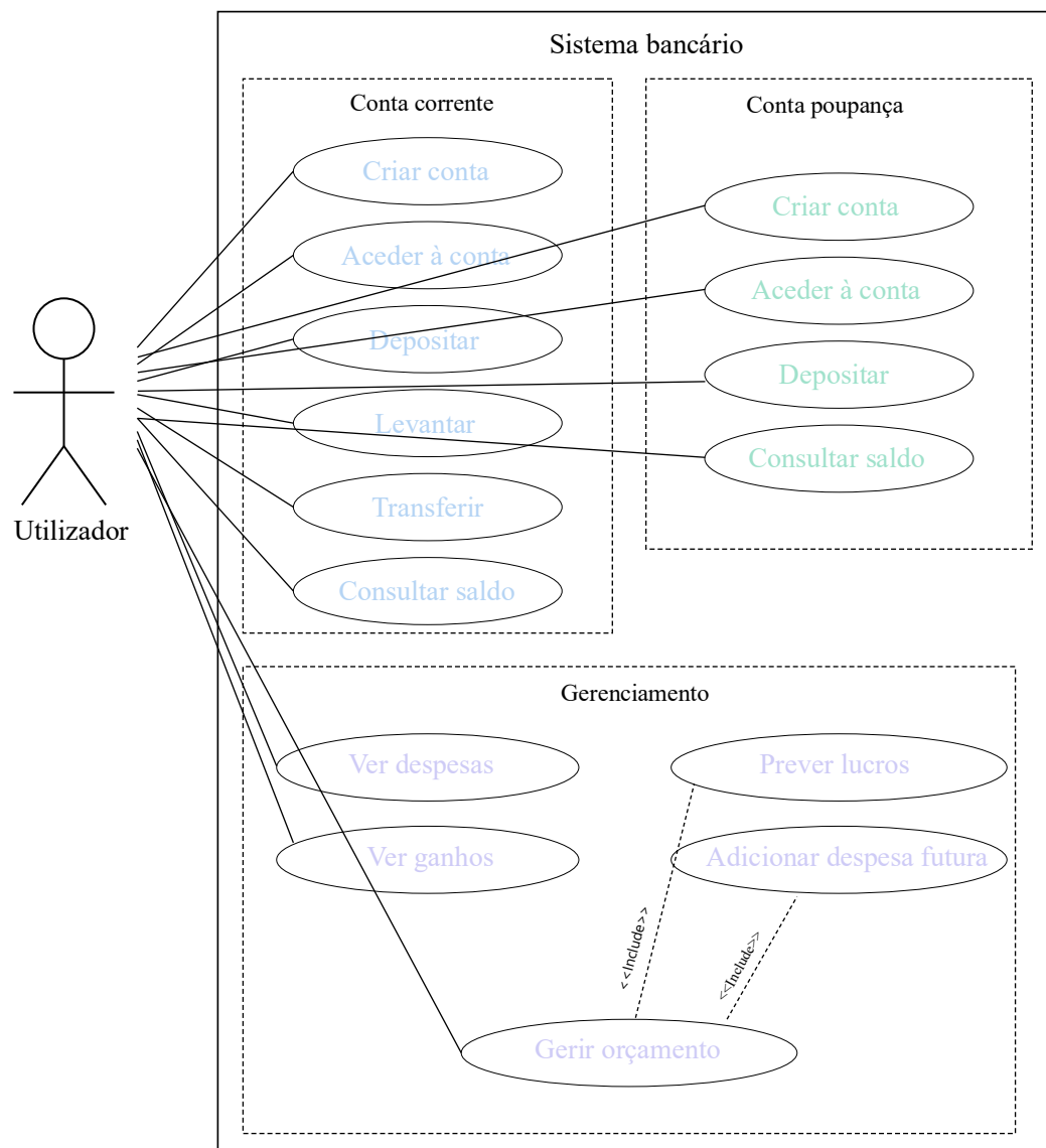
Figura 1 – Diagrama de Casos de Uso da Plataforma do Sistema Bancário
