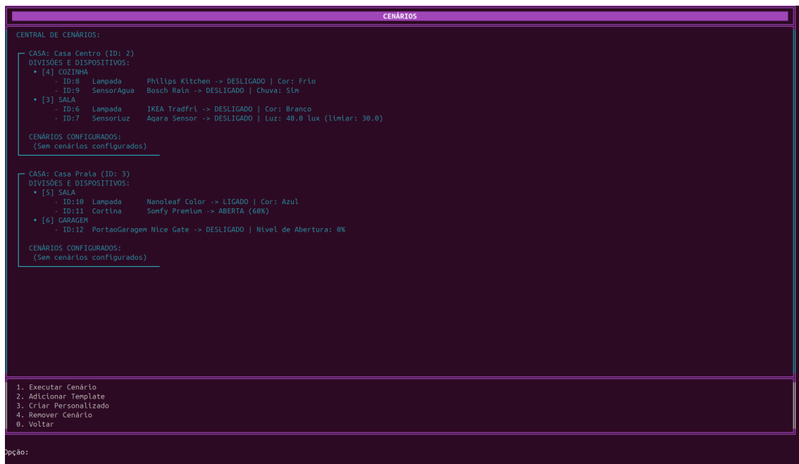
Figura 10: Menu Cenários
