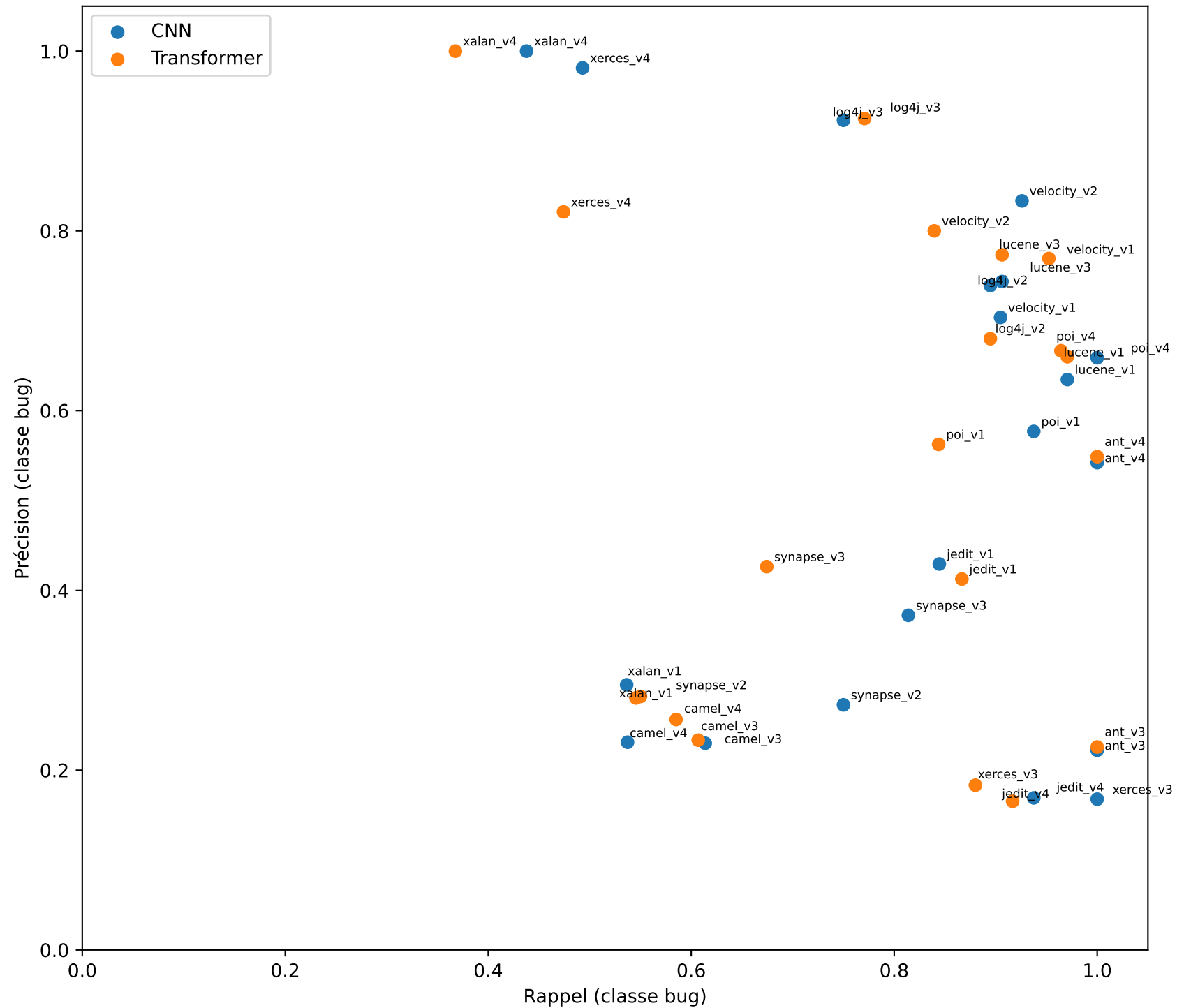
Compromis précision-rappel (F1)
