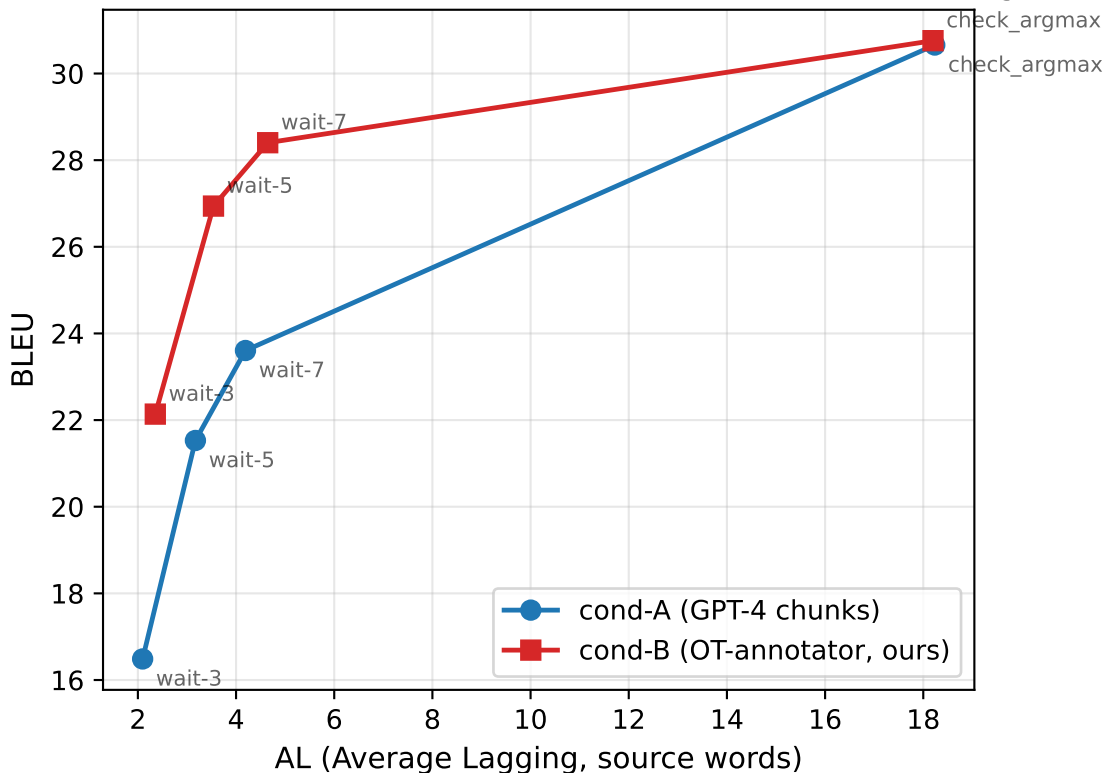
Gemma-4-E2B (n=10K) — newstest2013 De→En, streaming
