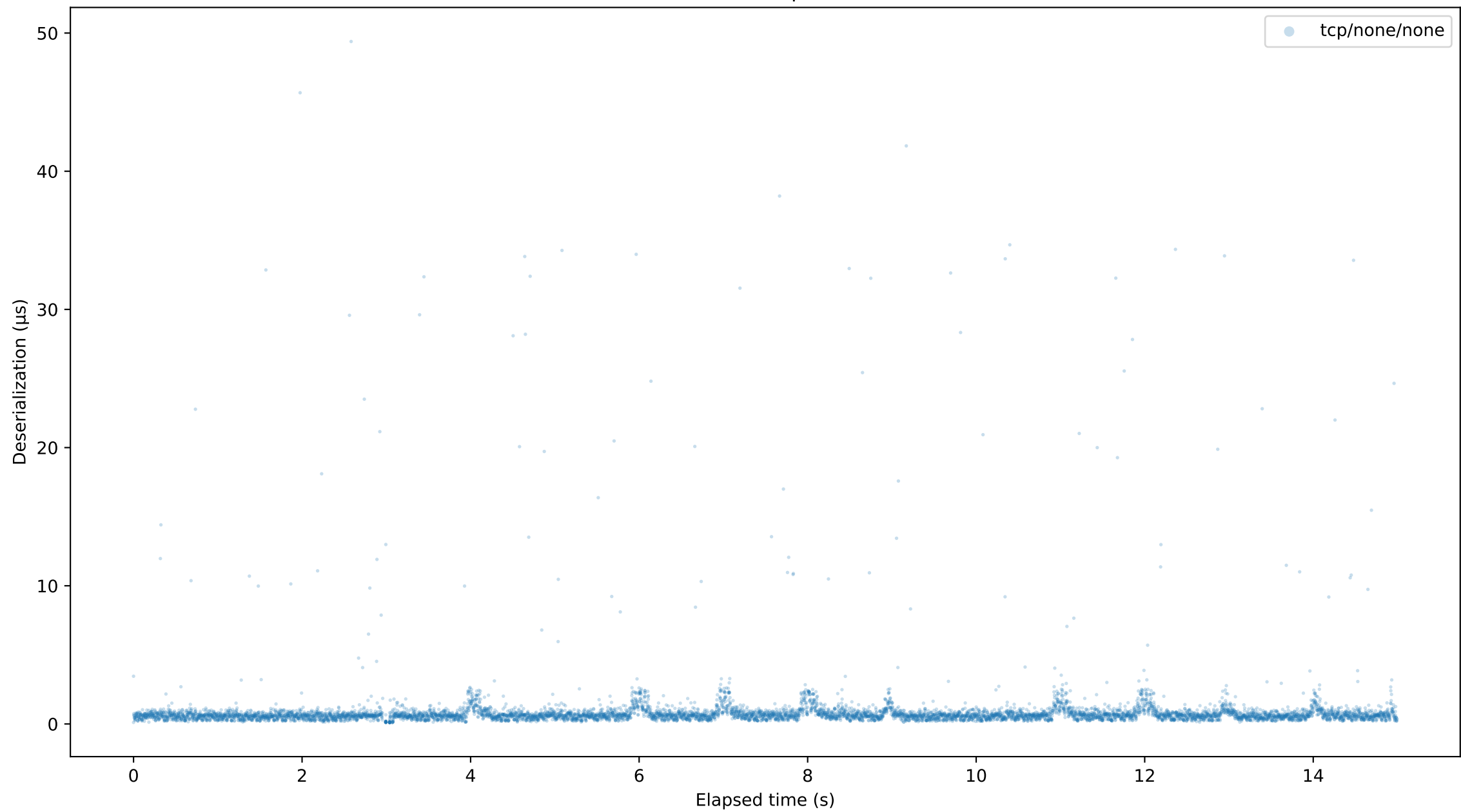
Deserialization per Packet
