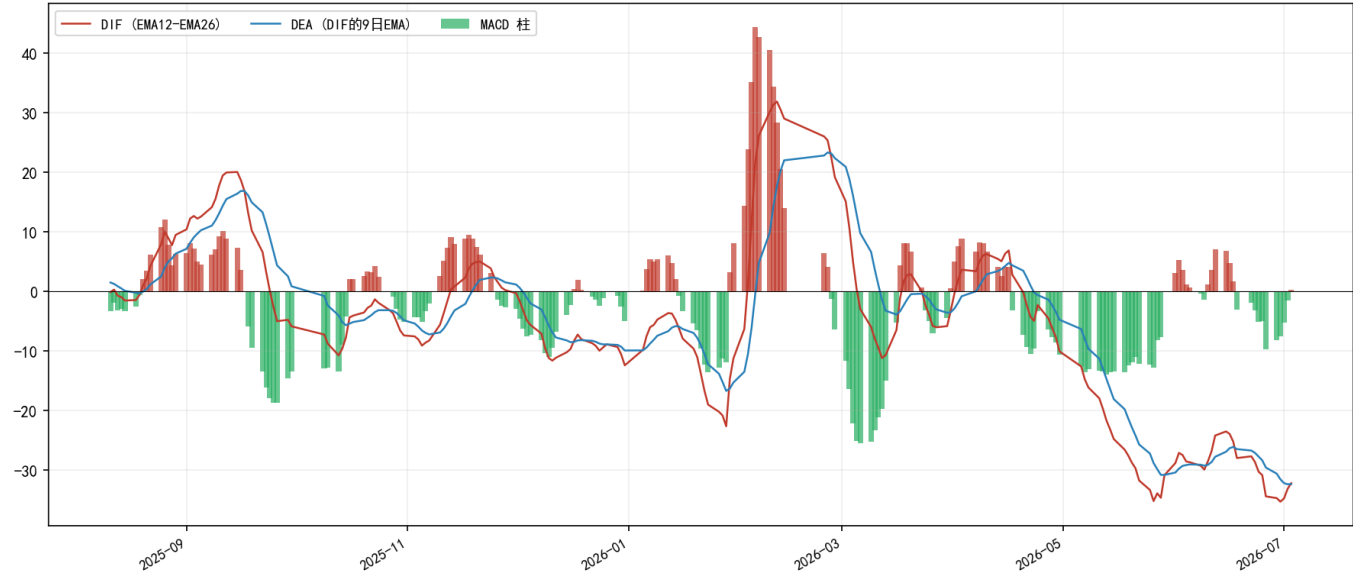
图 2：MACD (12, 26, 9)
