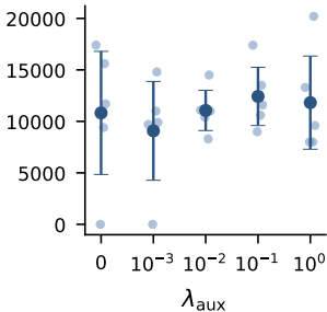
Grokking epoch
