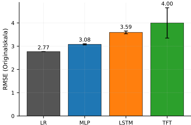
Test-RMSE — primäre Metrik
