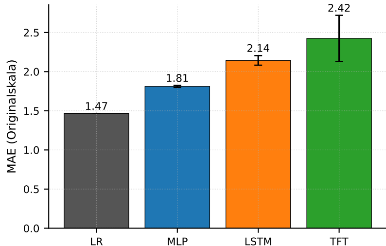
Test-MAE — sekundäre Metrik
