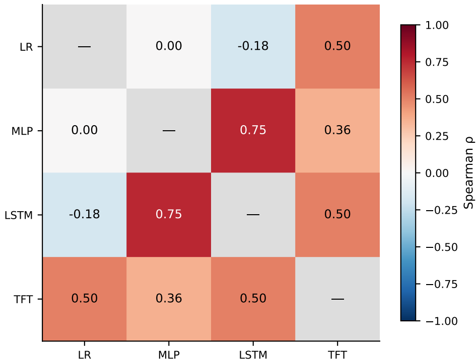
Modellübergreifende Rang-Übereinstimmung (Spearman \rho ) für Occlusion-Wichtigkeiten
