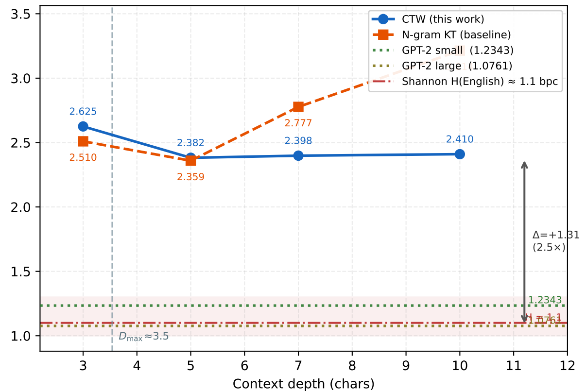
text8 (enwiki)
