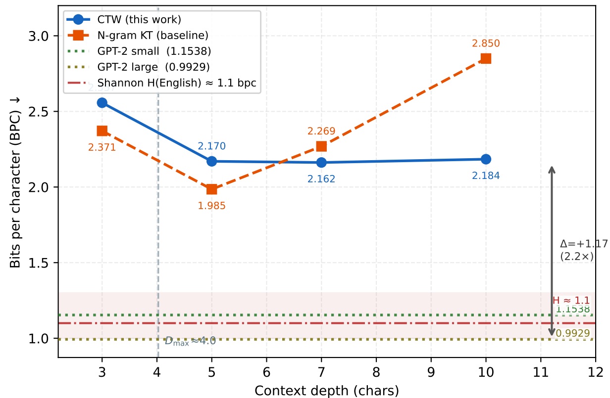
WikiText-2
