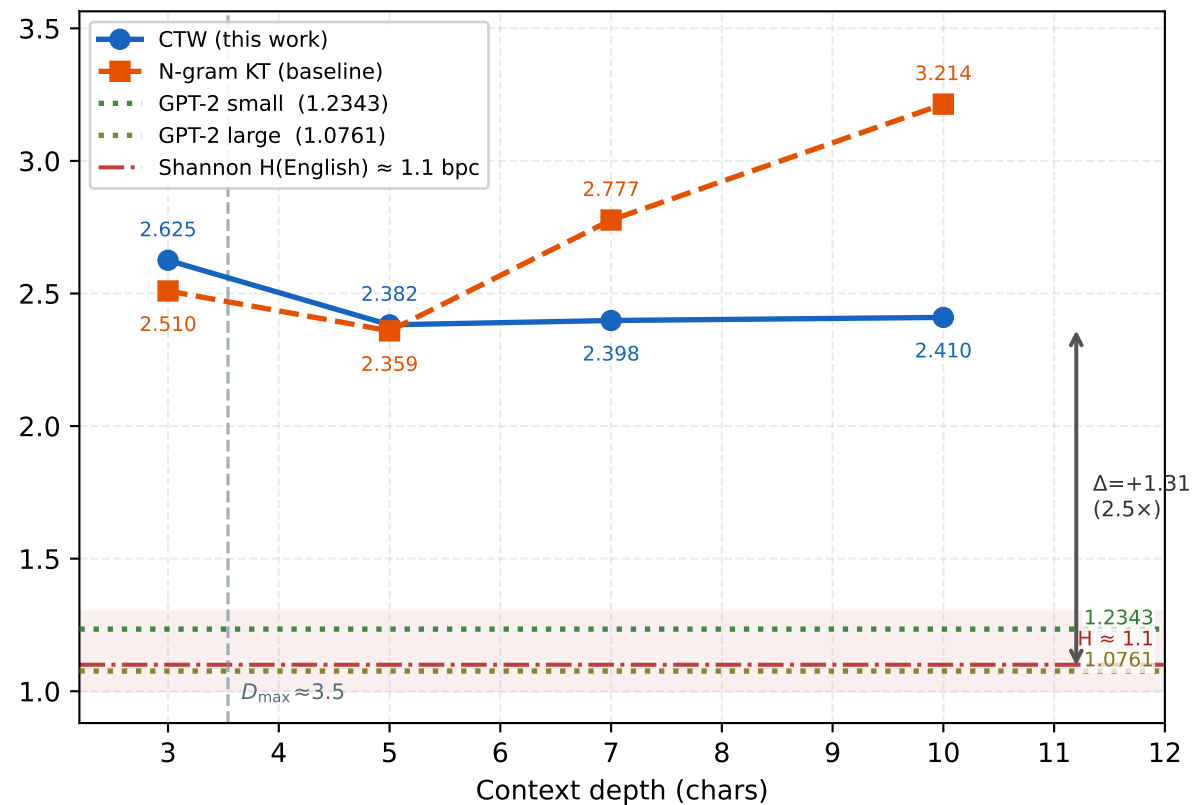
text8 (enwiki)
