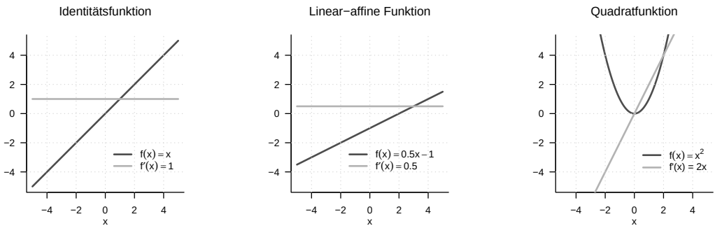
Abbildung 6.2 Ableitungen dreier elementarer Funktionen. Die Ableitung der Identitätsfunktion ist die konstante Funktion mit Wert 1, die Ableitung der betrachteten linear-affinen Funktion ist die konstante Funktion mit Wert 0.5 und die Ableitung der Quadratfunktion ist die linear-affine Funktion mit a = 2 und b = 0
