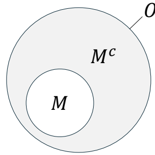
Abbildung 2.3 Venn-Euler-Diagramm des Komplements von M bezüglich O . Die grau hinterlegte Fläche entspricht M^c = O \setminus M .
