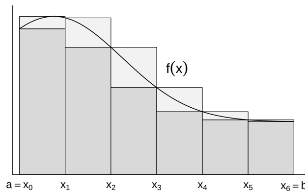
Abbildung 7.2 Zerlegung und Riemannsche Ober- und Untersummen
