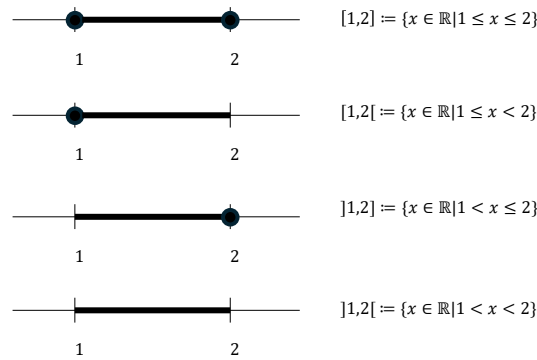
Abbildung 2.6 Darstellung von Intervallen am Zahlenstrahl. Der schwarze Punkt signalisiert dabei, dass die entsprechende Zahl Teil des Intervalls ist.
