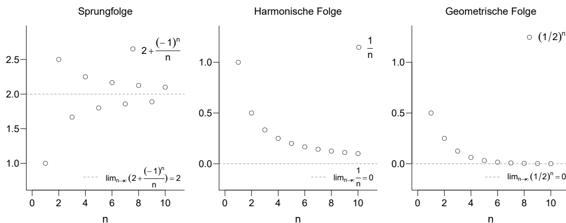
Abbildung 5.2 Grenzwerte der Sprungfolge, der harmonischen und der geometrischen Folge.
