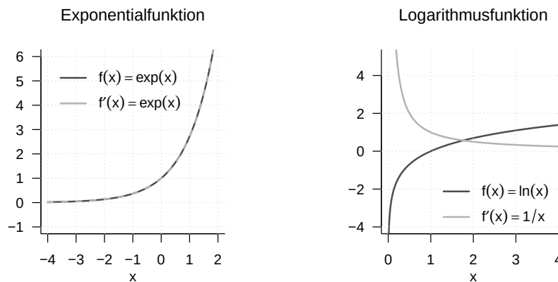
Abbildung 6.3 Ableitungen von Exponentialfunktion und Logarithmusfunktion. Die Ableitung der Exponentialfunktion ist die Exponentialfunktion selbst, die Ableitung der Logarithmusfunktion hat die Funktionswerte 1/x
