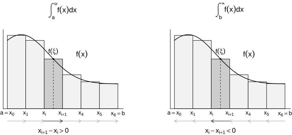
Abbildung 7.5 Orientierung bestimmter Integrale
