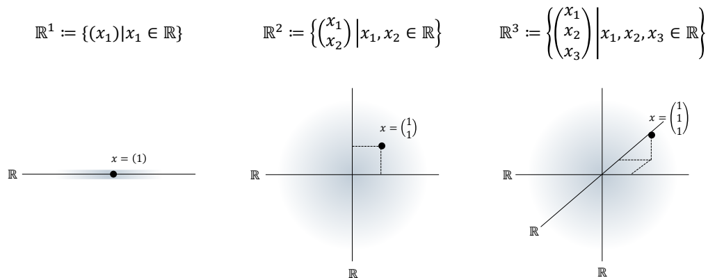
Abbildung 2.7 \mathbb{R}^n für n = 1, n = 2 und n = 3 . Die schwarzen Punkte stellen jeweils ein Element der entsprechenden Menge dar.
