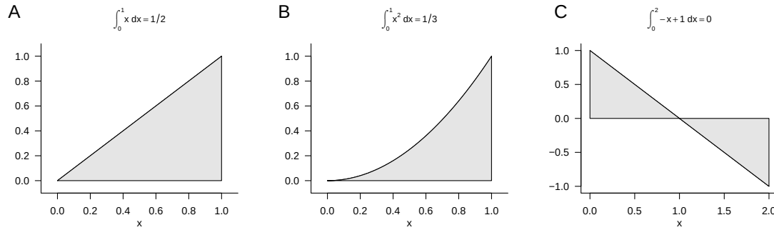
Abbildung 7.7 Beispiele zum Zweiten Hauptsatz der Differenzial- und Integralrechnung
