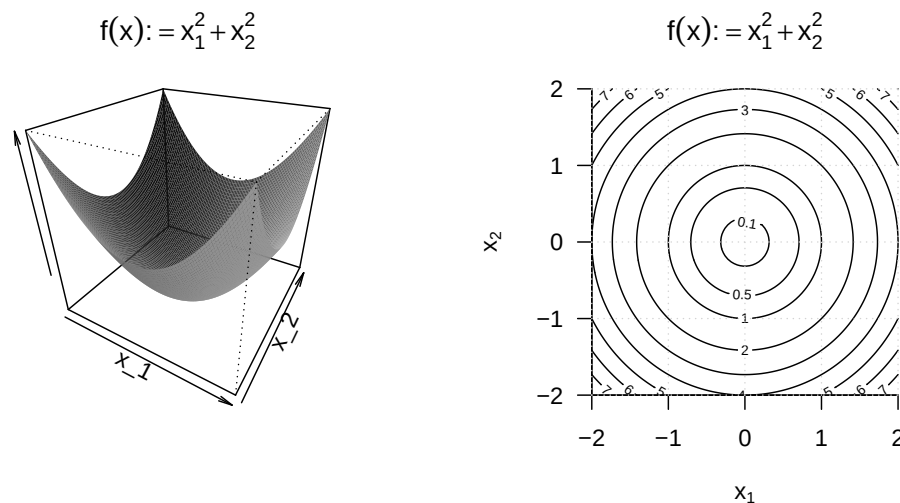
Abbildung 6.6 Visualisierungen einer bivariaten Funktion. Die linke Darstellung visualisiert die Funktionswerte als Fläche über der zweidimensionalen Definitionsmenge der Funktion. Auch wenn diese Darstellung einen gewissen dreidimensionalen Charakter hat, handelt es sich um eine bivariate Funktion mit entsprechend zweidimensionaler Definitionsmenge. Die rechte Abbildung visualisiert Linien mit gleichen Funktionswerten in der zweidimensionalen Definitionsmenge der Funktion.
