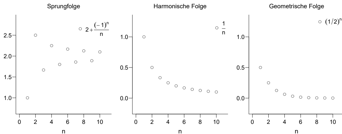
Abbildung 5.1 Sprungfolge, harmonische Folge und geometrische Folge ohne eingezeichnete Grenzwerte.
