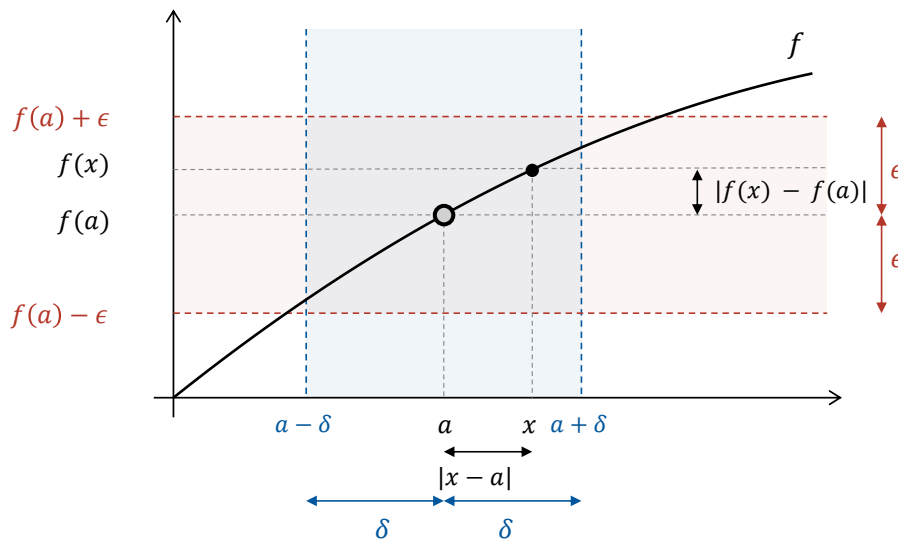
Abbildung 5.4 Zu jedem \epsilon > 0 lässt sich ein \delta > 0 so wählen, dass für alle x \in D aus |x - a| < \delta die Ungleichung |f(x) - f(a)| < \epsilon folgt.
