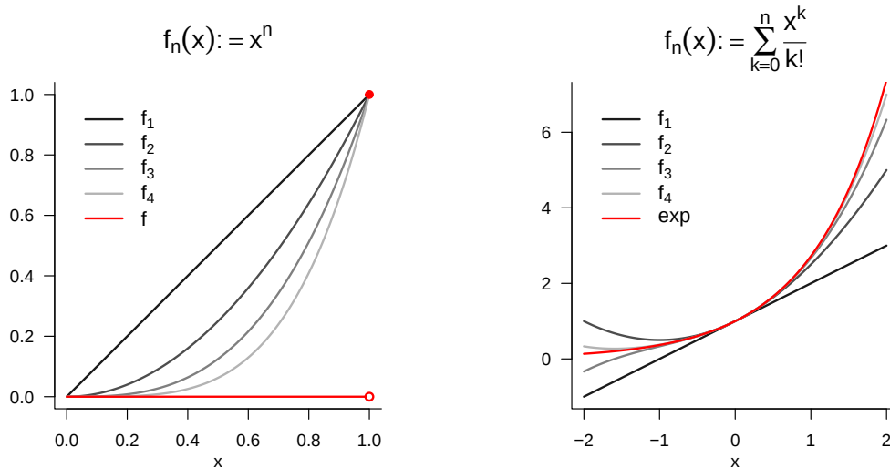
Abbildung 5.3 Beispiele für Grenzwerte von Funktionenfolgen
