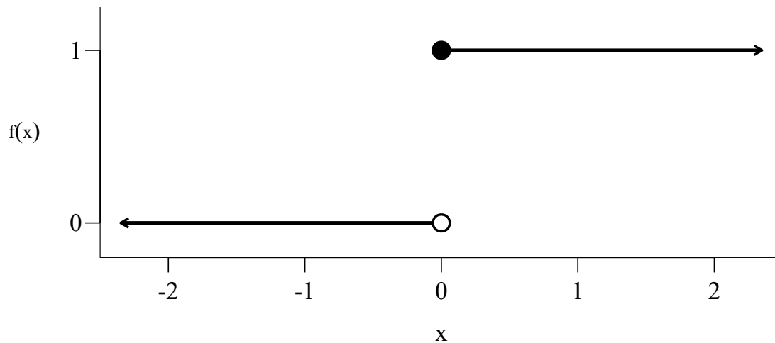
Abbildung 5.5 Heaviside-Funktion mit f(0) = 1 .
