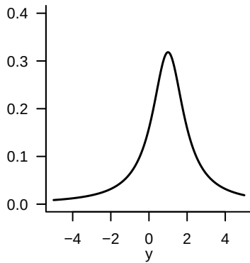
C(y;1,1)
