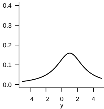
C(y;1,2)
