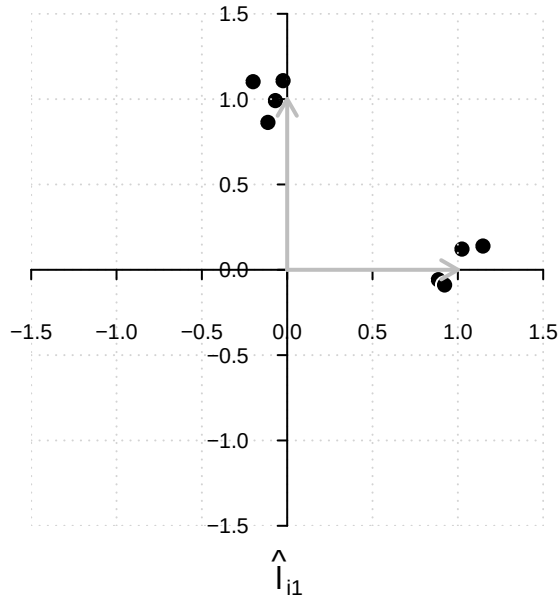
Einfachstruktur
