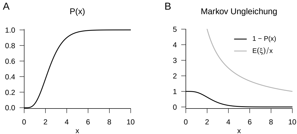
Abbildung 9.1 Markov-Ungleichung am Beispiel einer Gamma-Zufallsvariable.
