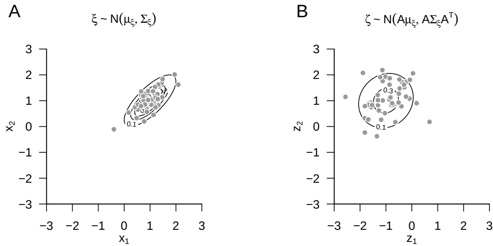
Abbildung 12.8 Invertierbare lineare Transformation eines normalverteilten Zufallsvektors
