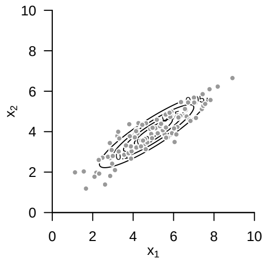
Abbildung 12.2 Konstruktion einer bivariaten Normalverteilung.
