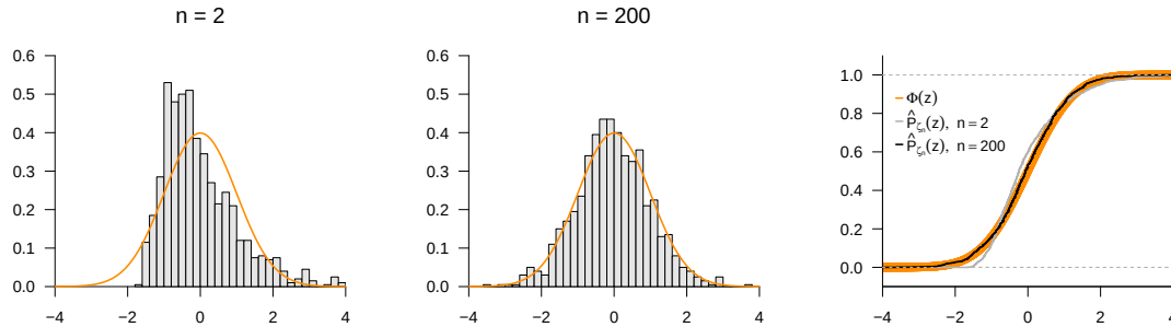
Abbildung 10.2 Simulation des Zentralen Grenzwertsatzes nach Lindeberg und Lévy.
