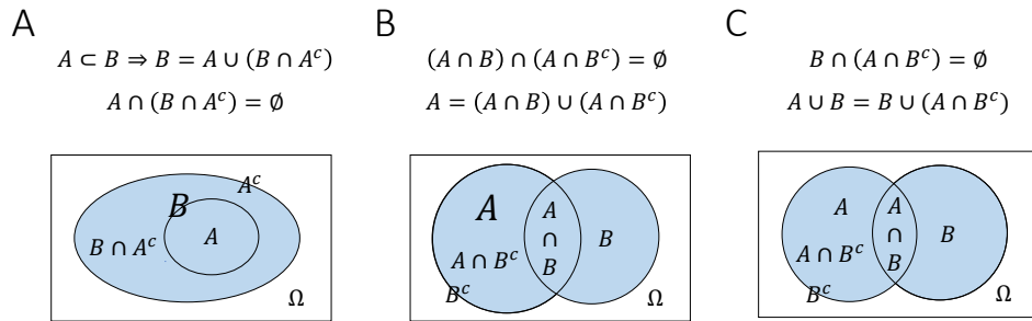
Abbildung 3.2 Venn-Diagramme zum Beweis von Theorem 3.1
