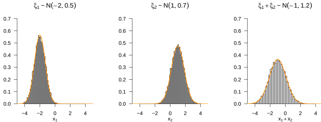
Abbildung 12.9 Summation normalverteilter Zufallsvariablen.
