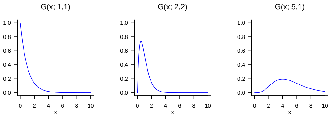
Abbildung 4.7 WDFen von Gamma-Zufallsvariablen.
