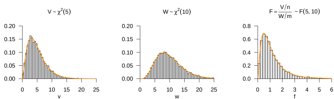
Abbildung 12.19 F -Transformation normalverteilter Zufallsvariablen.
