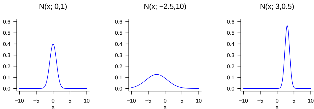
Abbildung 4.6 WDFen von normalverteilten Zufallsvariablen.
