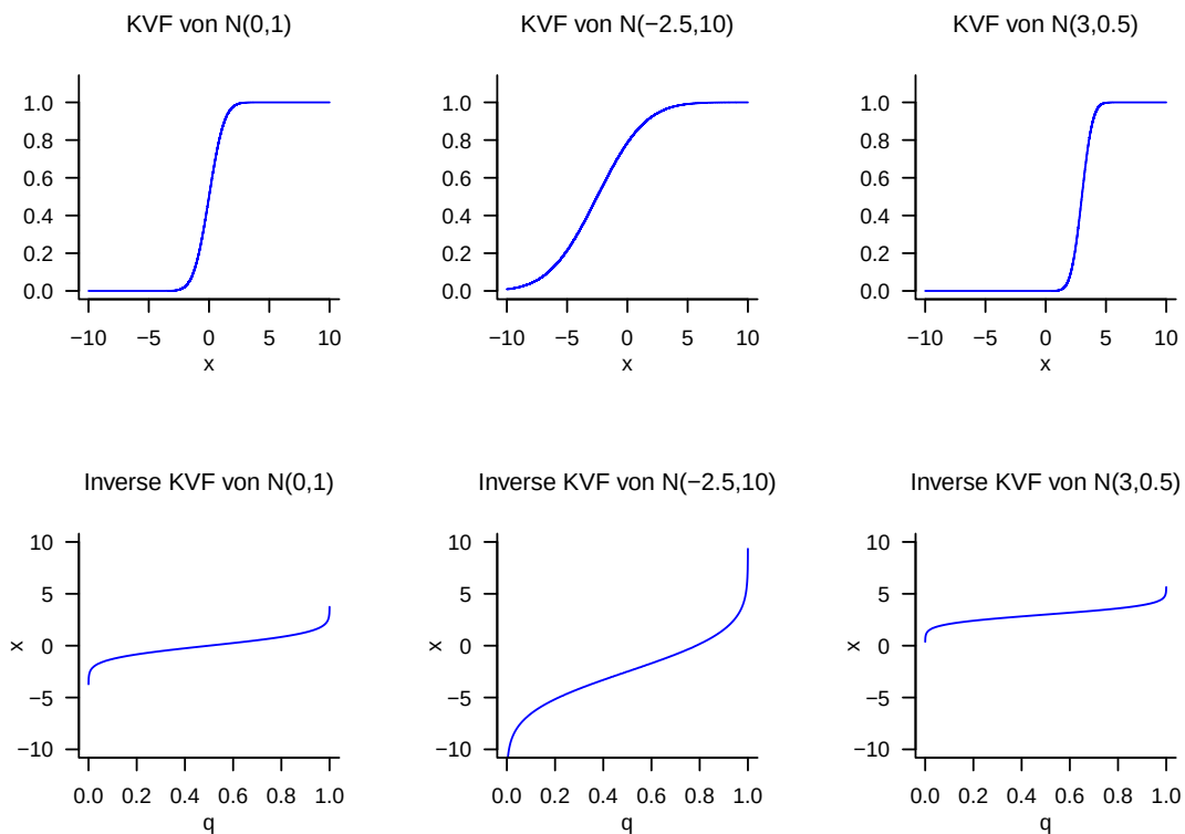
Abbildung 4.13 KVFe und inverse KVFe von normalverteilten Zufallsvariablen.
