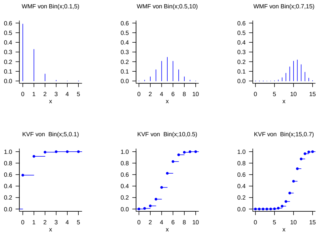
Abbildung 4.11 WMFen und KVFen von Binomial-Zufallsvariablen.
