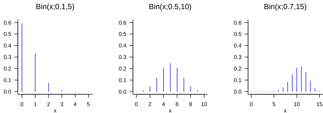
Abbildung 4.4 WMFen von Binomial-Zufallsvariablen.
