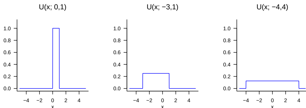
Abbildung 4.9 WDFen von gleichverteilten-Zufallsvariablen.
