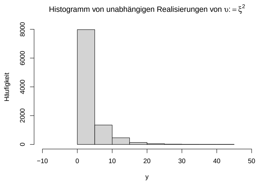
Abbildung 11.2 Histogramm von 10.000 quadrierten Realisierungen unabhängig und identisch normalverteilter Zufallsvariablen.
