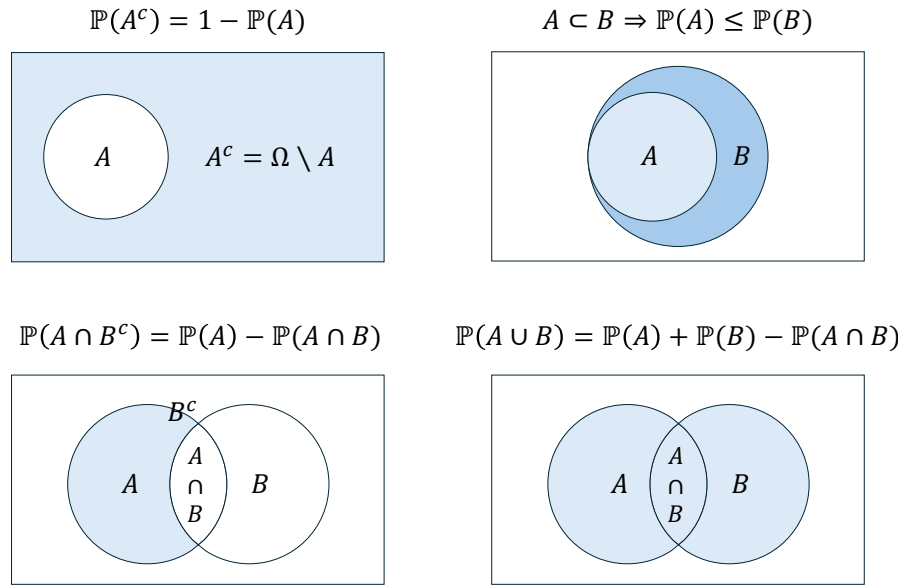
Abbildung 3.1 Venn-Diagramme zu Theorem 3.1. Die hellblau unterlegten Flächen entsprechen jeweils den Wahrscheinlichkeiten von Interesse
