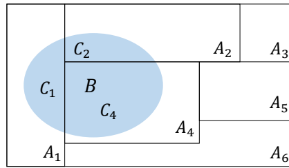
Abbildung 3.3 Venn-Diagramm zum Beweis von Theorem 3.4.
