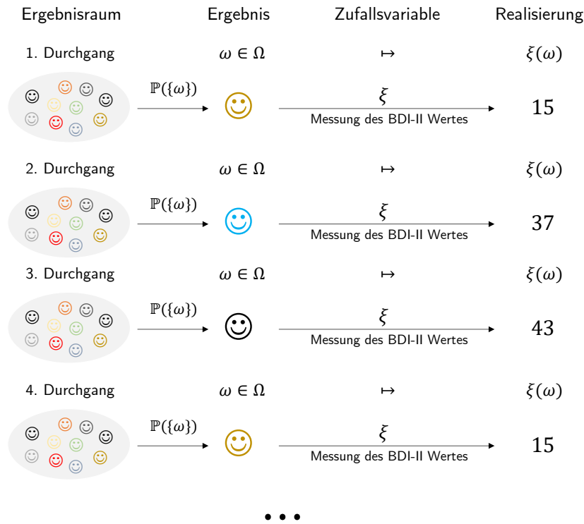
Abbildung 4.2 Zufallsvariable als Modell eines Messvorgangs.
