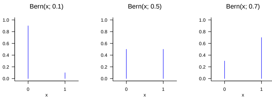
Abbildung 4.3 WMFen von Bernoulli-Zufallsvariablen.
