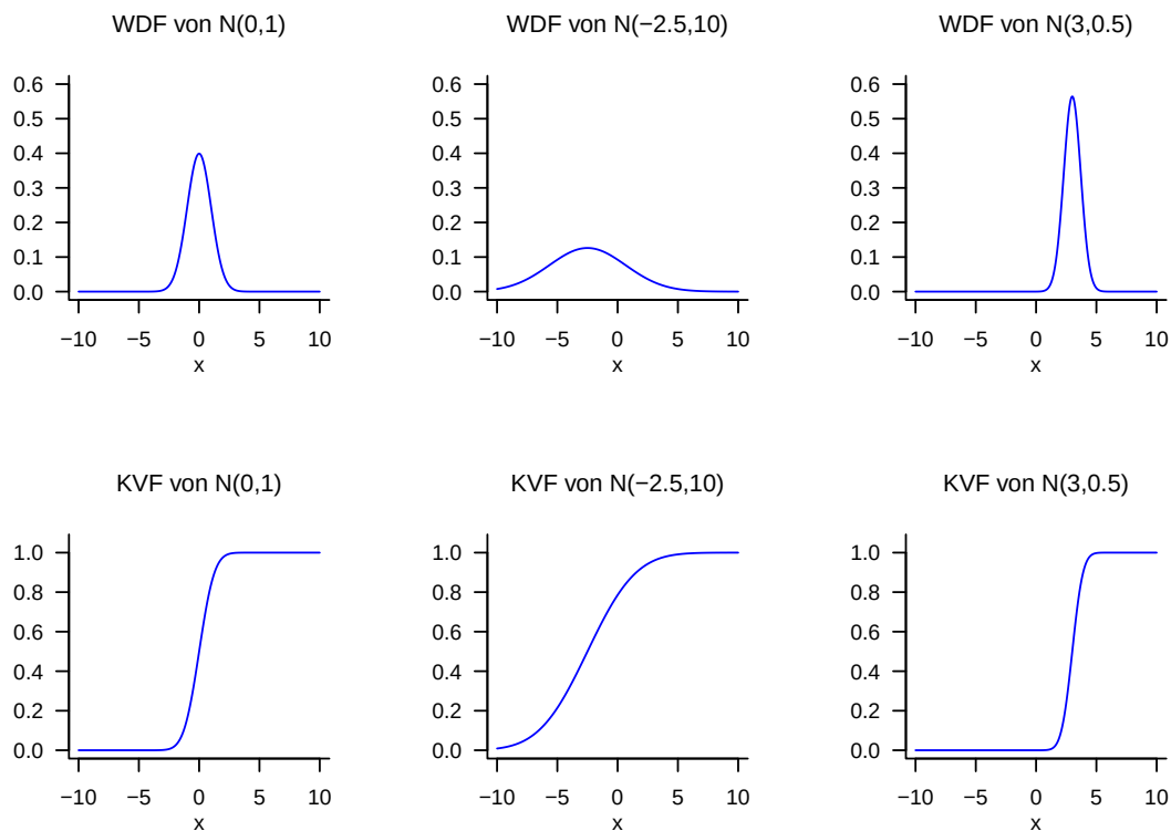
Abbildung 4.12 WDFen und KVFe von normalverteilten Zufallsvariablen.
