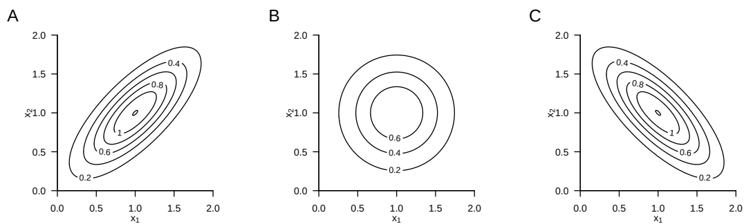
Abbildung 12.3 Wahrscheinlichkeitsdichtefunktionen bivariater Normalverteilungen.
