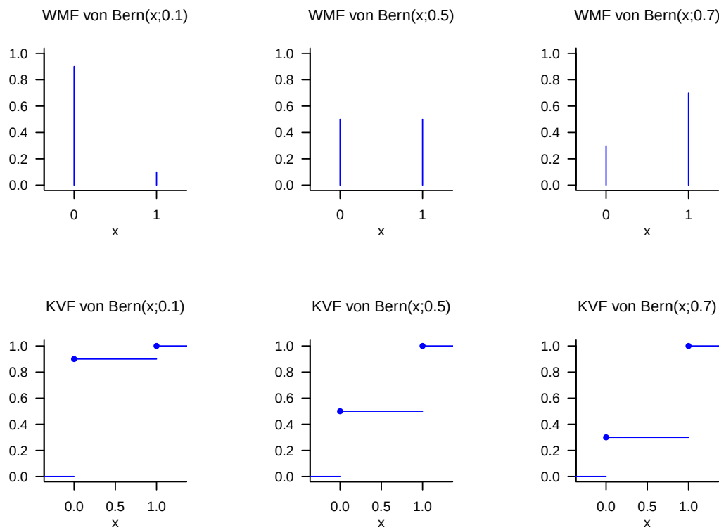
Abbildung 4.10 WMFen und KVFen von Bernoulli-Zufallsvariablen.
