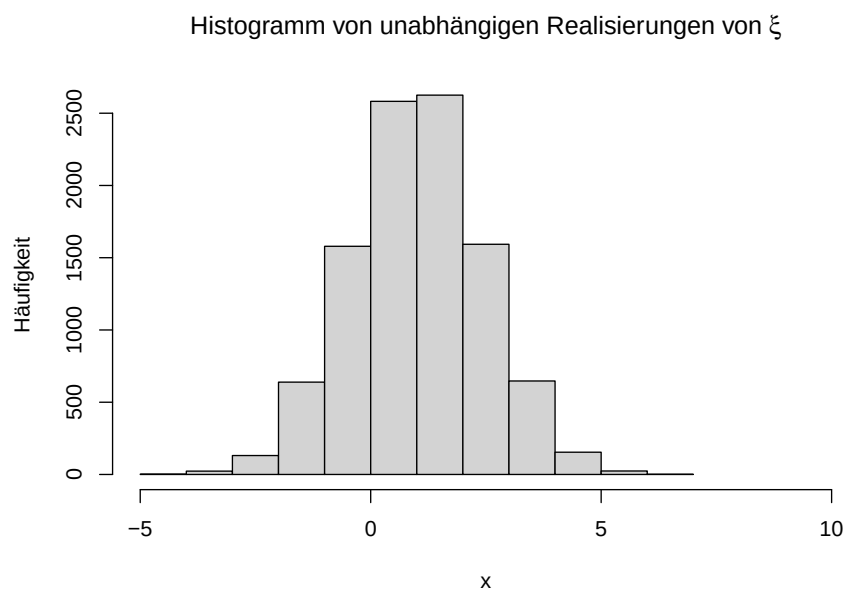
Abbildung 11.1 Histogramm von 10.000 Realisierungen unabhängig und identisch normalverteilter Zufallsvariablen.
