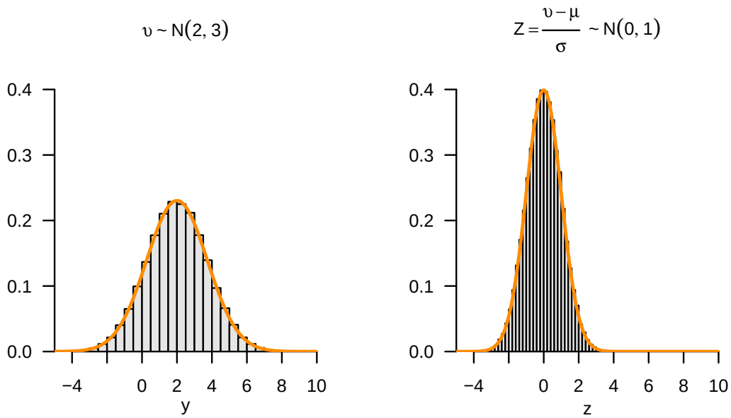
Abbildung 12.11 Z-Transformation normalverteilter Zufallsvariablen.
