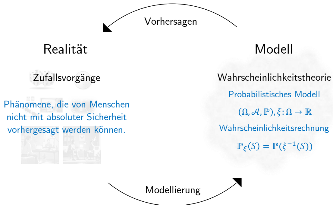
Abbildung 1.1 Wahrscheinlichkeitstheorie als Modell von Zufallsvorgängen. Ausgangspunkt der Wahrscheinlichkeitstheorie ist die Absicht, über einen Zufallsvorgang, also ein mit Unsicherheit behaftetes Phänomen der Wirklichkeit, logisch-quantitative Schlüsse zu ziehen. Die Repräsentation zentraler Aspekte des Zufallsvorgangs mithilfe wahrscheinlichkeitstheoretischer Begrifflichkeiten bezeichnet man als Modellierung . Das wahrscheinlichkeitstheoretische Modell selbst garantiert dann im Sinne der Wahrscheinlichkeitsrechnung die Korrektheit logisch-quantitativer Schlussfolgerungen, welche zur Vorhersage von Aspekten des Zufallsvorgangs genutzt werden können.
