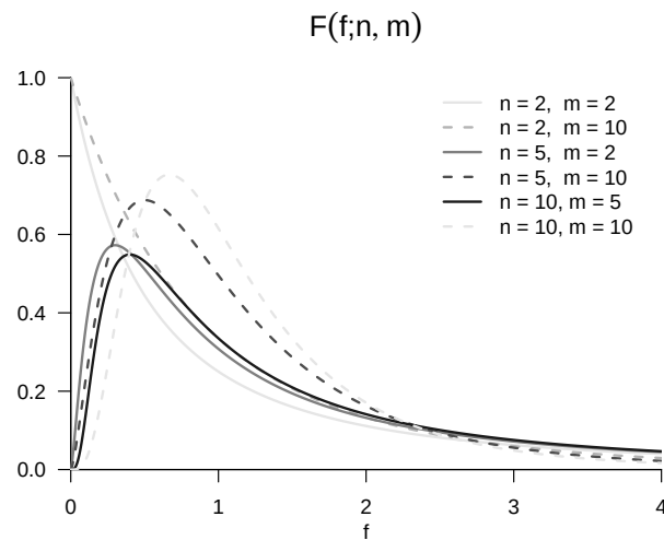
Abbildung 12.18 WDFen von F -verteilten Zufallsvariablen.
