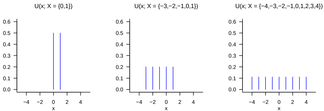
Abbildung 4.5 WMFen von diskret-gleichverteilten Zufallsvariablen.
