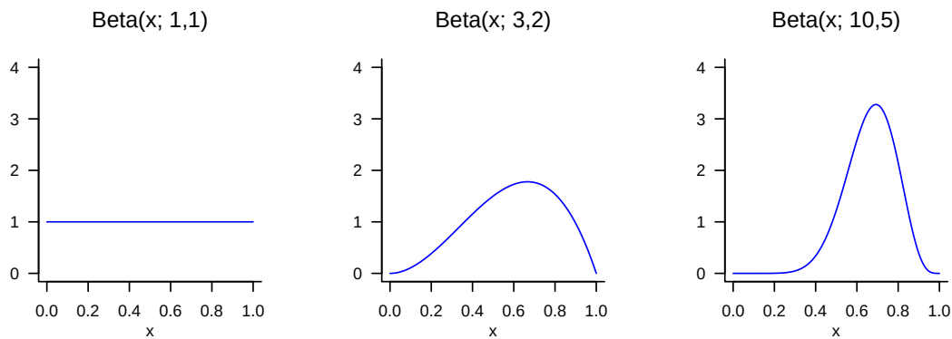
Abbildung 4.8 WDFen von Beta-Zufallsvariablen.
