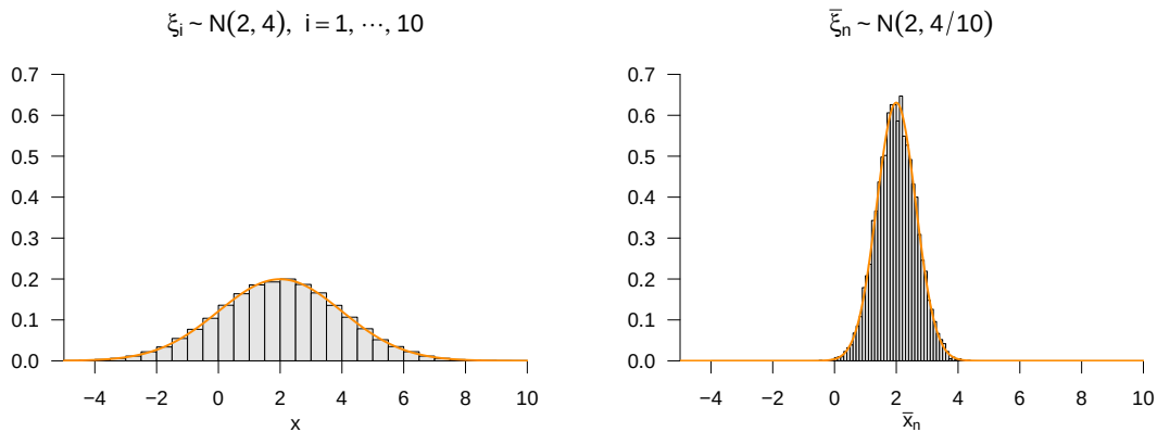
Abbildung 12.10 Mittelwertbildung bei normalverteilten Zufallsvariablen.
