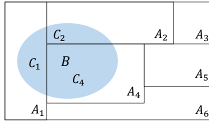
Abbildung 14.2. Venn-Diagramm zum Beweis von Theorem 14.3.
