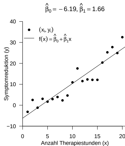
Abbildung 28.4. Ausgleichsgerade für den Beispieldatensatz.
