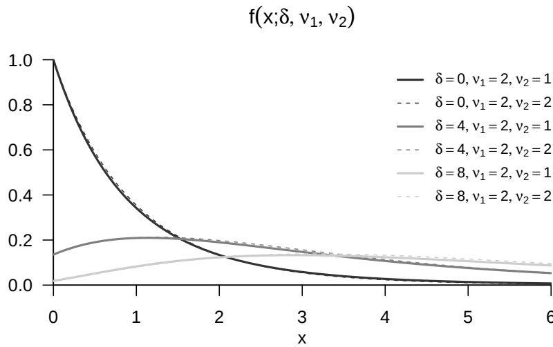
Abbildung 40.3. Exemplarische WDFen einer nichtzentralen f -Zufallsvariable
