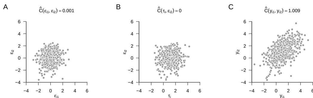
Abbildung 44.3. Normalverteilungsbeispiel bezüglich zweier paralleler Testmessungen.
