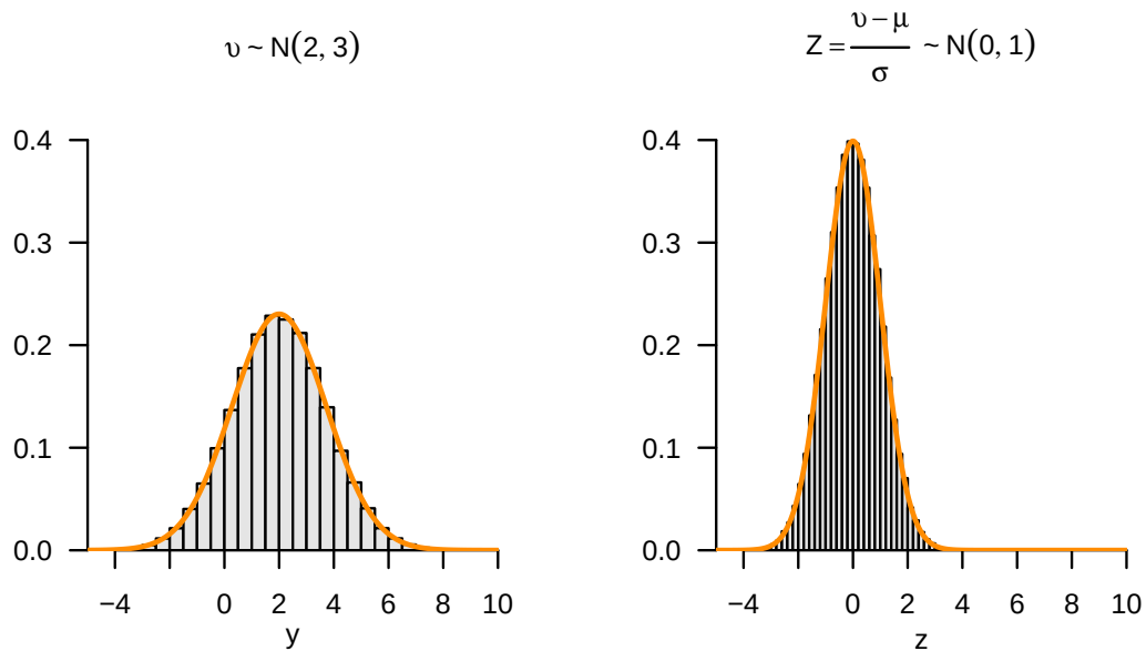
Abbildung 23.11. Z -Transformation normalverteilter Zufallsvariablen.
