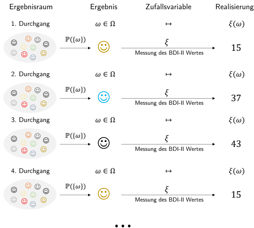
Abbildung 15.2. Zufallsvariable als Modell eines Messvorgangs.
