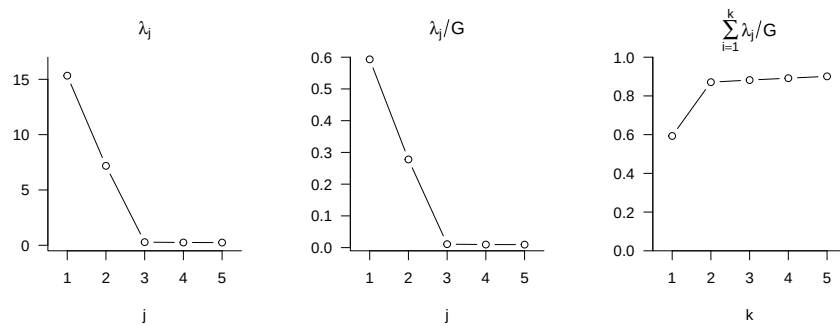
Abbildung 45.5. Scree-Plot und relative und kumulative Gesamtstichprobenvarianz durch steigende Faktorenanzahlen für den BDI-II Datensatz nach Keller et al. (2008).
