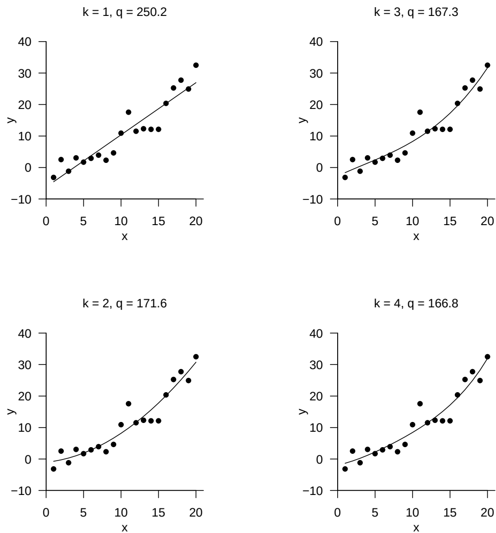
Abbildung 28.5. Ausgleichspolynome ersten bis vierten Grades für den Beispieldatensatz.
