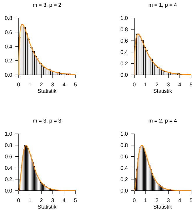
Abbildung 41.3. Simulation spezieller Verteilungen der Wilks'- \Lambda -Statistik Transformationen bei Zutreffen der Nullhypothese.
