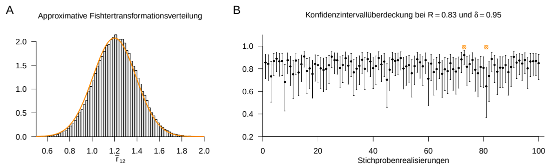
Abbildung 44.4. A Simulation der Verteilung der Fisher-transformierten Stichprobenkorrelation und ihre analytische Approximation B Simulation der Überdeckungswahrscheinlichkeit des Konfidenzintervalls für die Stichprobenkorrelation bei einer wahren, aber unbekannten, Korrelation von R = 0.833 und einer gewünschten Überdeckungswahrscheinlichkeit von \delta := 0.95 . Die Abbildung zeigt für jede Stichprobenrealisierung das Konfidenzintervall und die entsprechende Stichprobenkorrelation. In der vorliegenden Simulation überdecken die Konfidenzintervalle, die durch eine graue Linie eingezeichnete immer gleichen wahren, aber unbekannten, Korrelation R := 0.833 in 98 von 100 Fällen. Die Stichprobenrealisierungen, für die dies nicht der Fall ist, sind mit einem orangefarbenen Kreis markiert.
