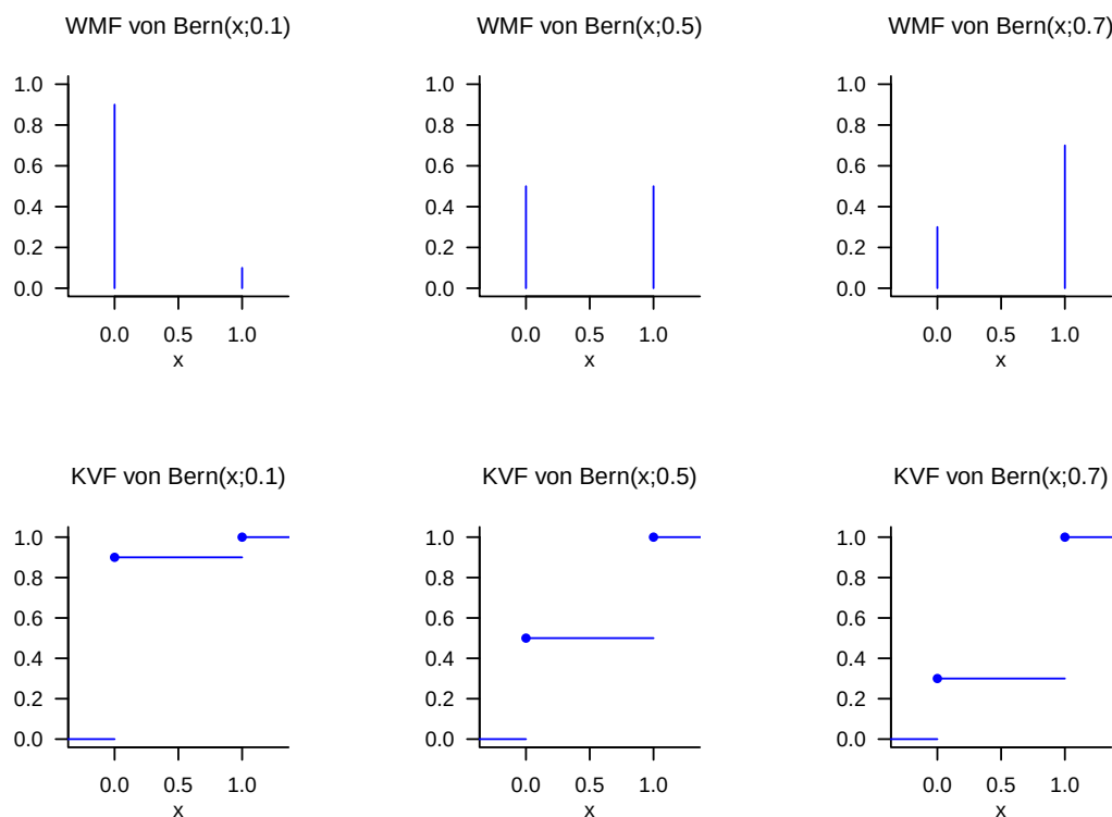
Abbildung 15.10. WMFen und KVFen von Bernoulli-Zufallsvariablen.
