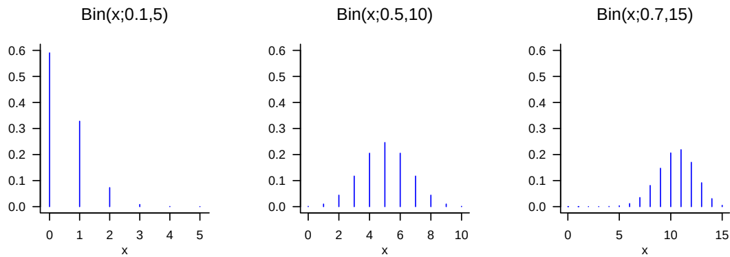
Abbildung 15.4. WMFen von Binomial-Zufallsvariablen.
