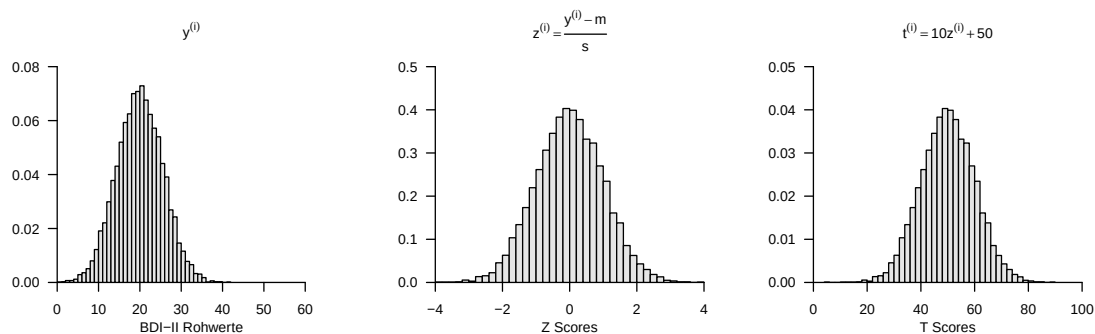
Abbildung 43.2. Simulierte Stichproben-BDI-II Rohwerte, Z Scores und T Scores
