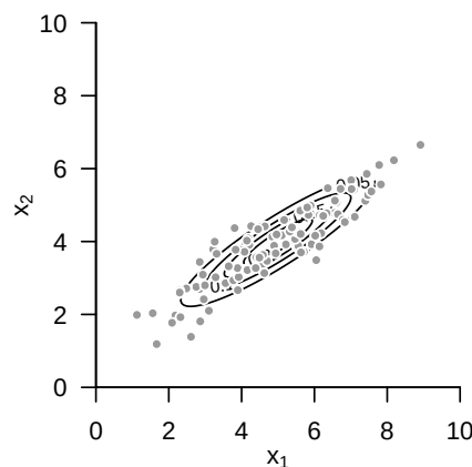
Abbildung 23.2. Konstruktion bivariater Normalverteilungen.
