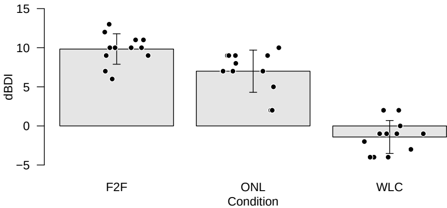
Abbildung 35.1. Datendarstellung des Anwendungsbeispiels zur Einfaktoriellen Varianzanalyse.
