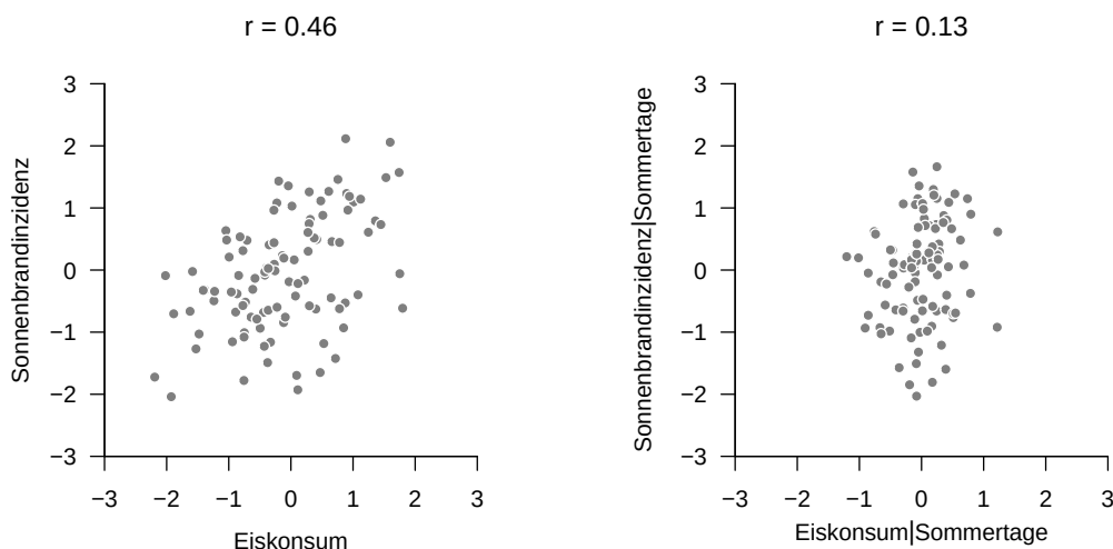
Abbildung 37.3. Evaluation der partiellen Korrelation im Beispielszenario.
