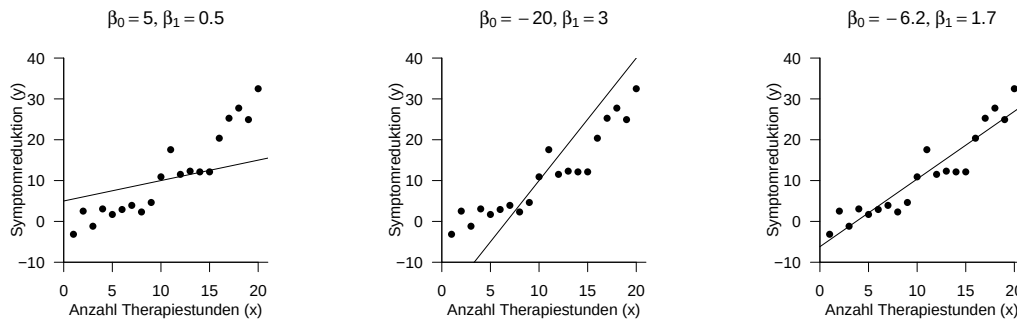
Abbildung 28.2. Linear-affine Funktionen mit unterschiedlichen Parameterwerten vor dem Hintergrund des Beispieldatensatzes.
