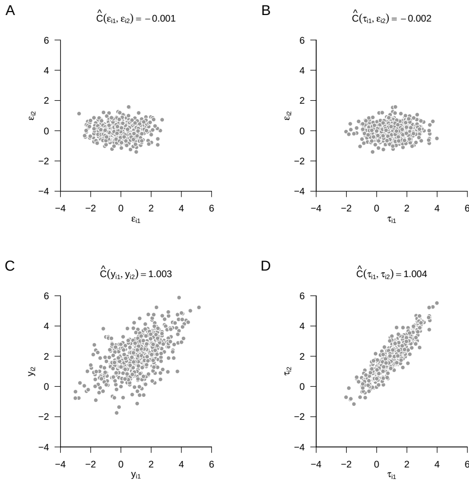
Abbildung 44.2. Normalverteilungsbeispiel bezüglich zweier Testmessungen.
