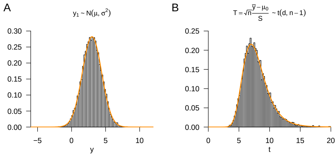
Abbildung 27.2. Verteilung der Einstichproben-T-Test-Statistik für n = 12 , \mu = 3 , \sigma^2 und \mu_0 = 0 . (A) Verteilung der Stichprobenvariablen. (B) Verteilung der Einstichproben-T-Test-Statistik
