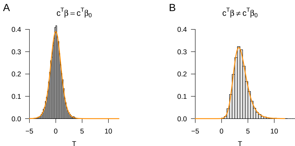
Abbildung 32.1. Verteilungen der T-Statistik bei unabhängig und identisch normalverteilten Zufallsvariablen.
