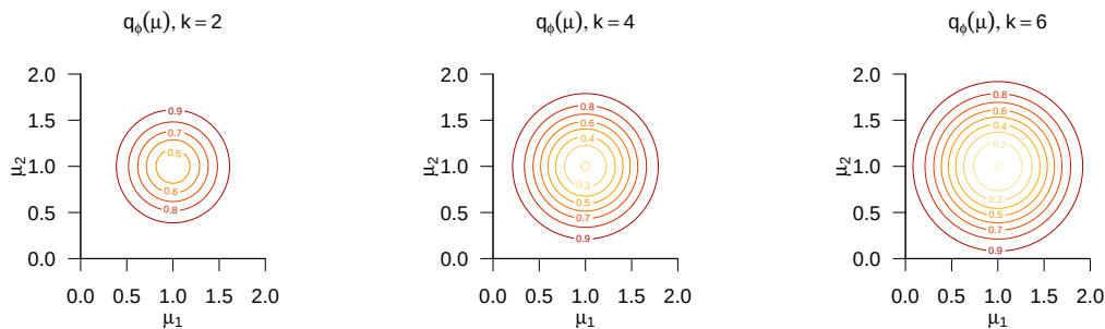
Abbildung 40.5. Einstichproben- T^2 -Test Testgütefunktionen für kritische Werte k = 2 , k = 4 und k = 6 im Szenario
