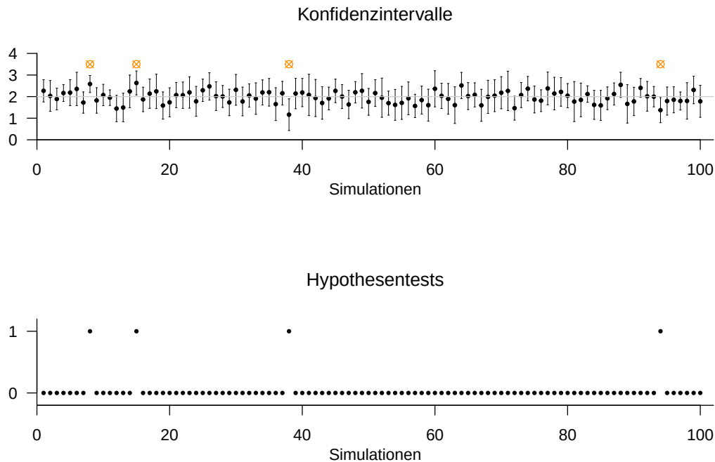
Abbildung 27.9. Dualität von Konfidenzintervall und Hypothesentest am Beispiel des Normalverteilungsmodells. Nutzt man das \delta -Konfidenzintervall für den Erwartungswertparameter um bei Nichtüberdeckung des Nullhypotheseparameters die Nullhypothese abzulehnen, so ergibt sich in diesem Fall ein Hypothesentest mit Signifikanzlevel \alpha_0 = 1 - \delta .
